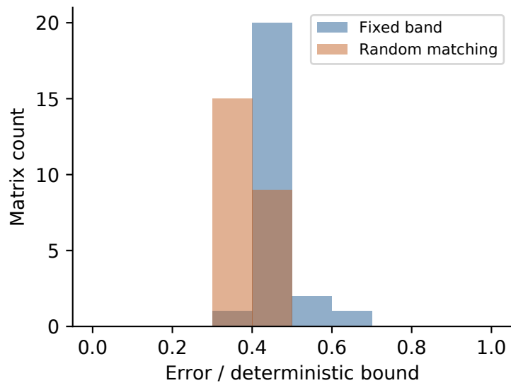
(b) N=64 , L=4 , time=1, r=4
