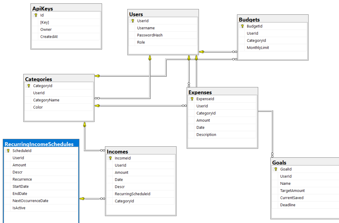
Figura 2 - Diagrama ER
