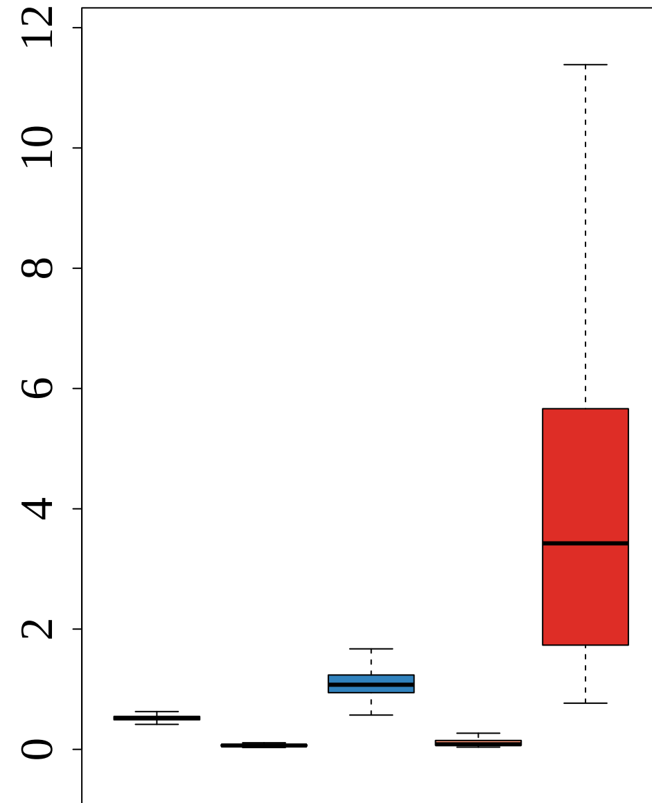
Posterior var.
