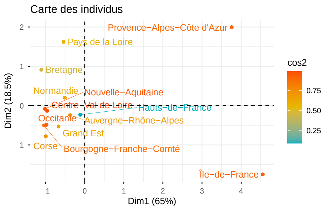
Graphique 26 : Projection des régions sur le plan
