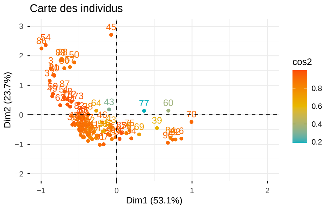
Graphique 23 : Zoom sur la projection des départements sur le plan
