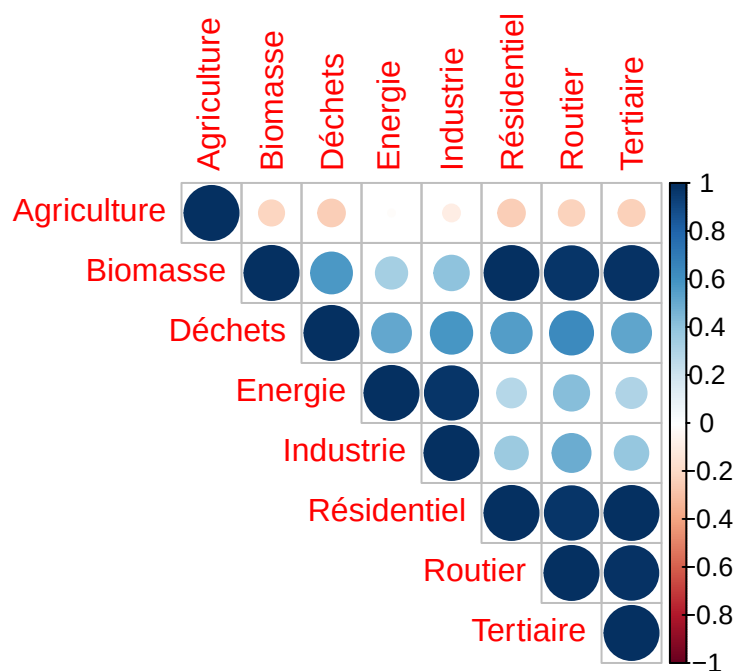
Graphique 7 : Corrélations des émissions de CO2 par secteur (Pearson)
