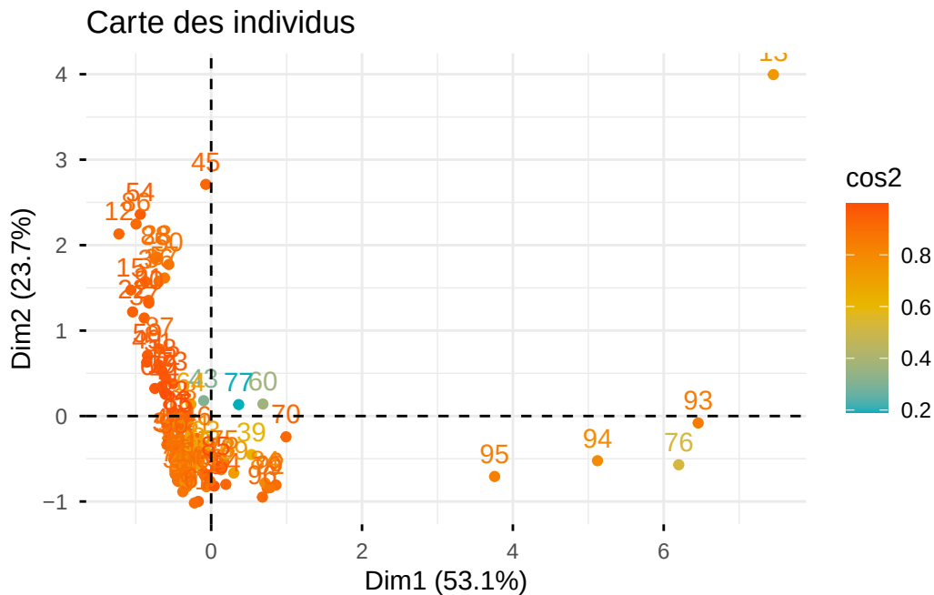
Graphique 22 : Projection des départements sur le plan
