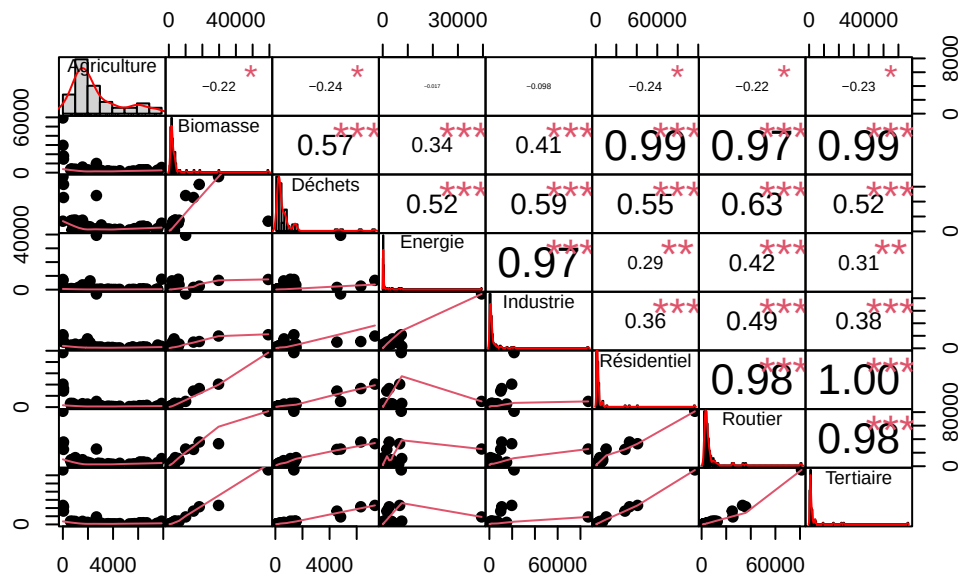
Graphique 6 : Corrélation des émissions de CO2 par secteur (Pearson)
