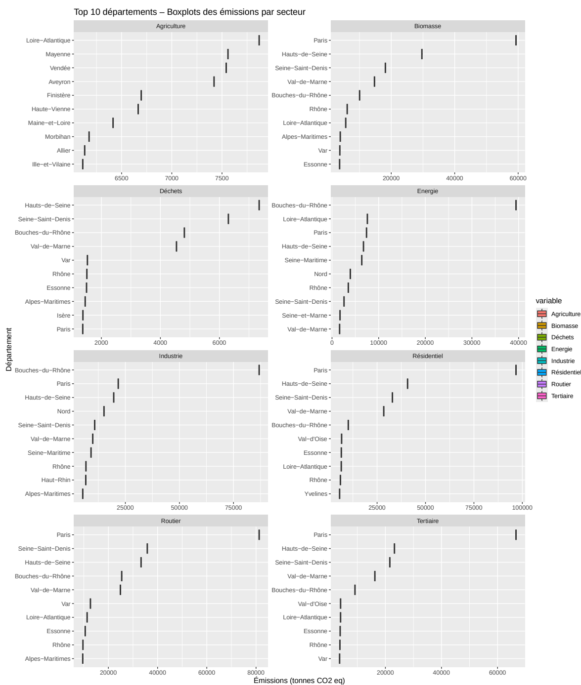
Graphique 13 : Top 10 des départements les plus émetteurs par secteurs
