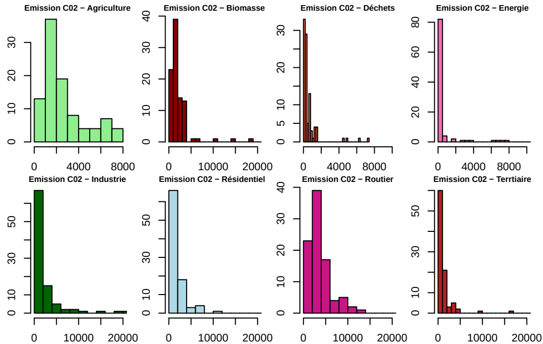
Graphiques 3 : Histogrammes zoomés des variables quantitatives
