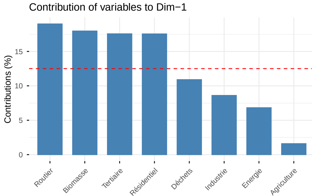
Graphique 16 : Contribution des variables à la première composante principale
