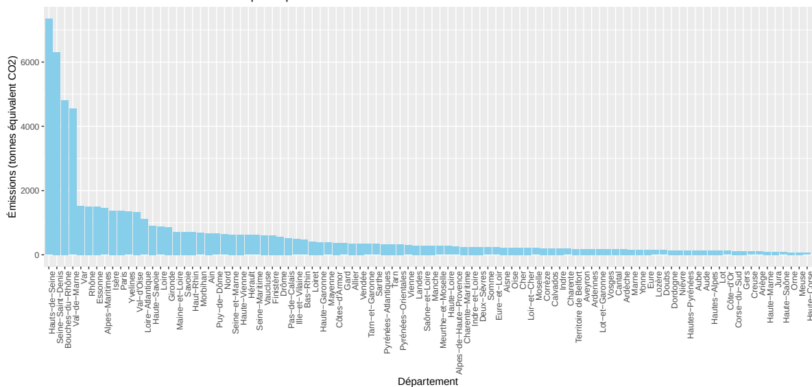
Émissions de CO2 – secteur Déchets par département
