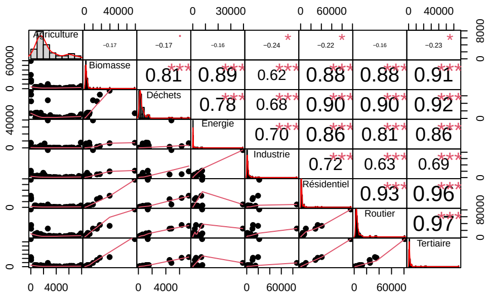
Graphique 8 : Corrélation des émissions de CO2 par secteur (Spearman)
