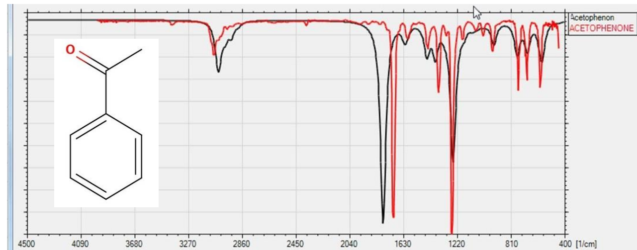
アセトフェノン分子の赤外吸収スペクトル
