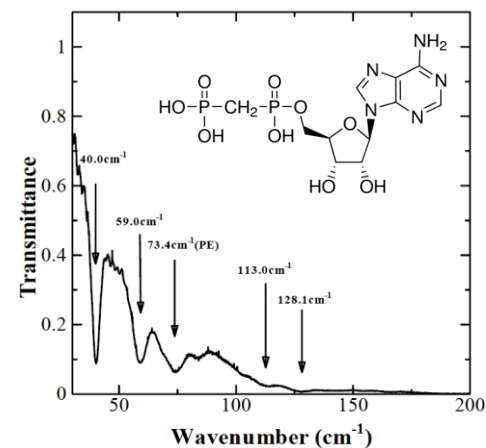
理研, THz database 2.0
