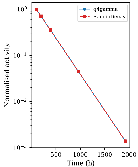
I131→I131
