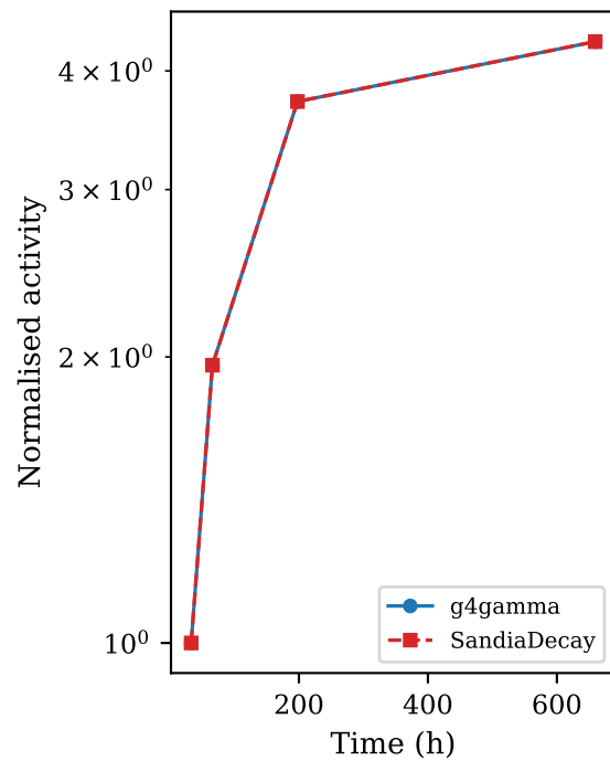
Mo99→Tc99
