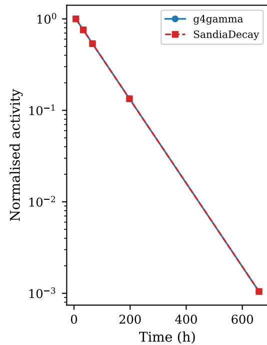
Mo99→Mo99
