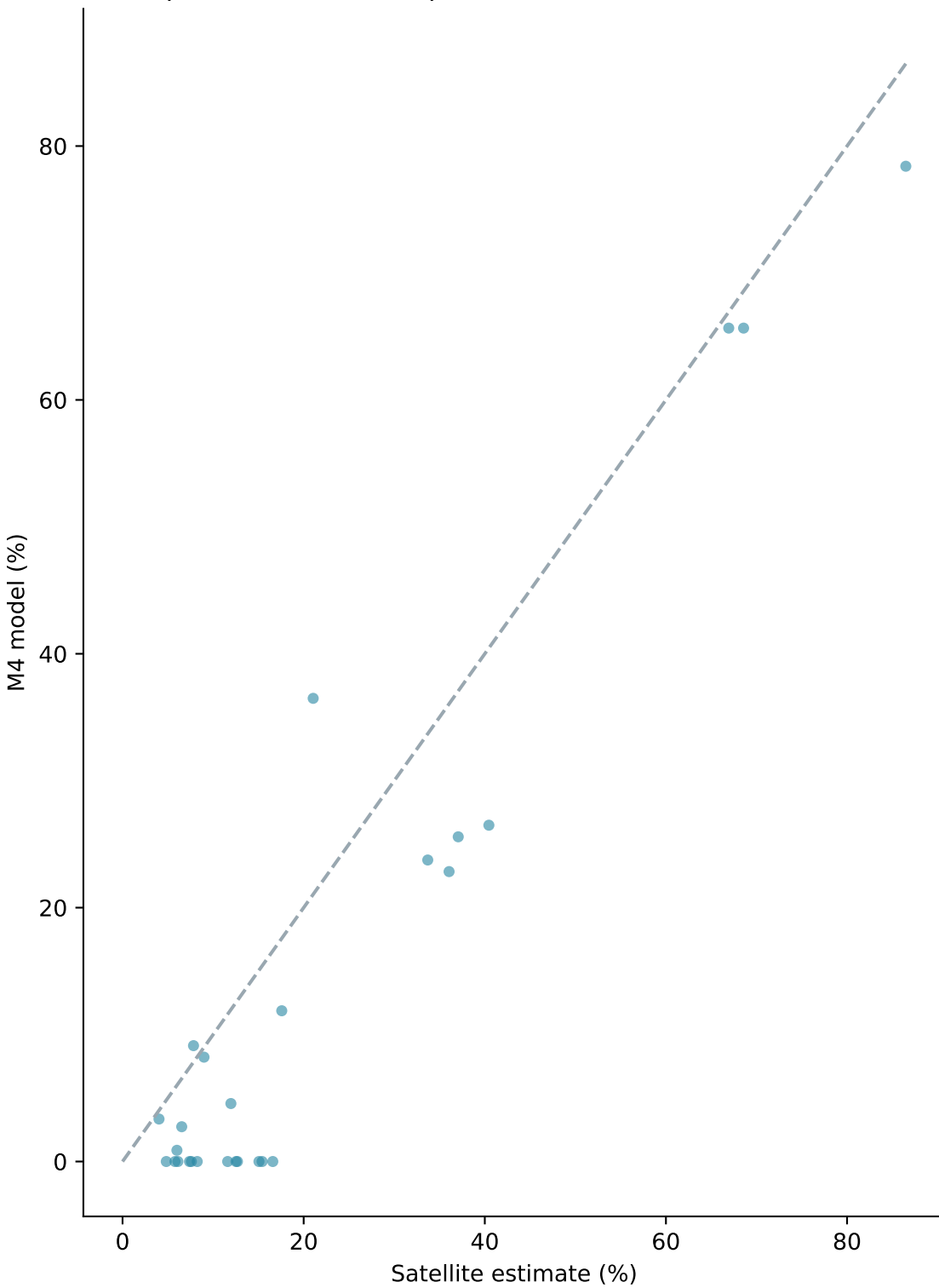
Snow process check · 27 pairs
