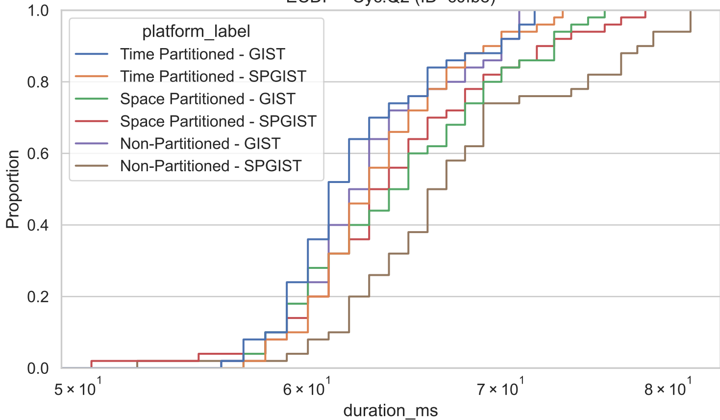
ECDF – Cyc.Q2 (ID=c0fbe)
