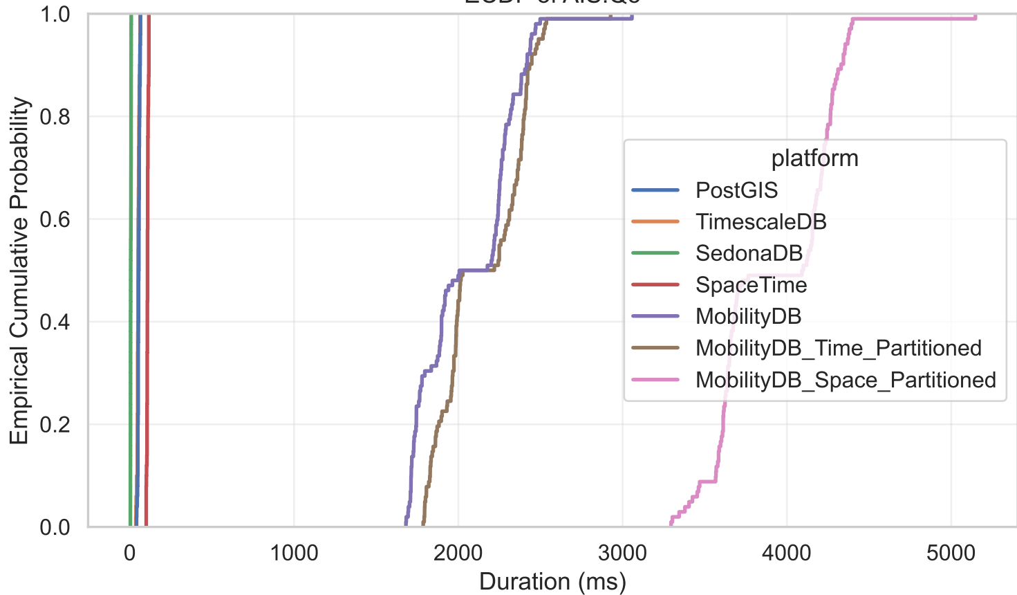
ECDF of AIS.Q5
