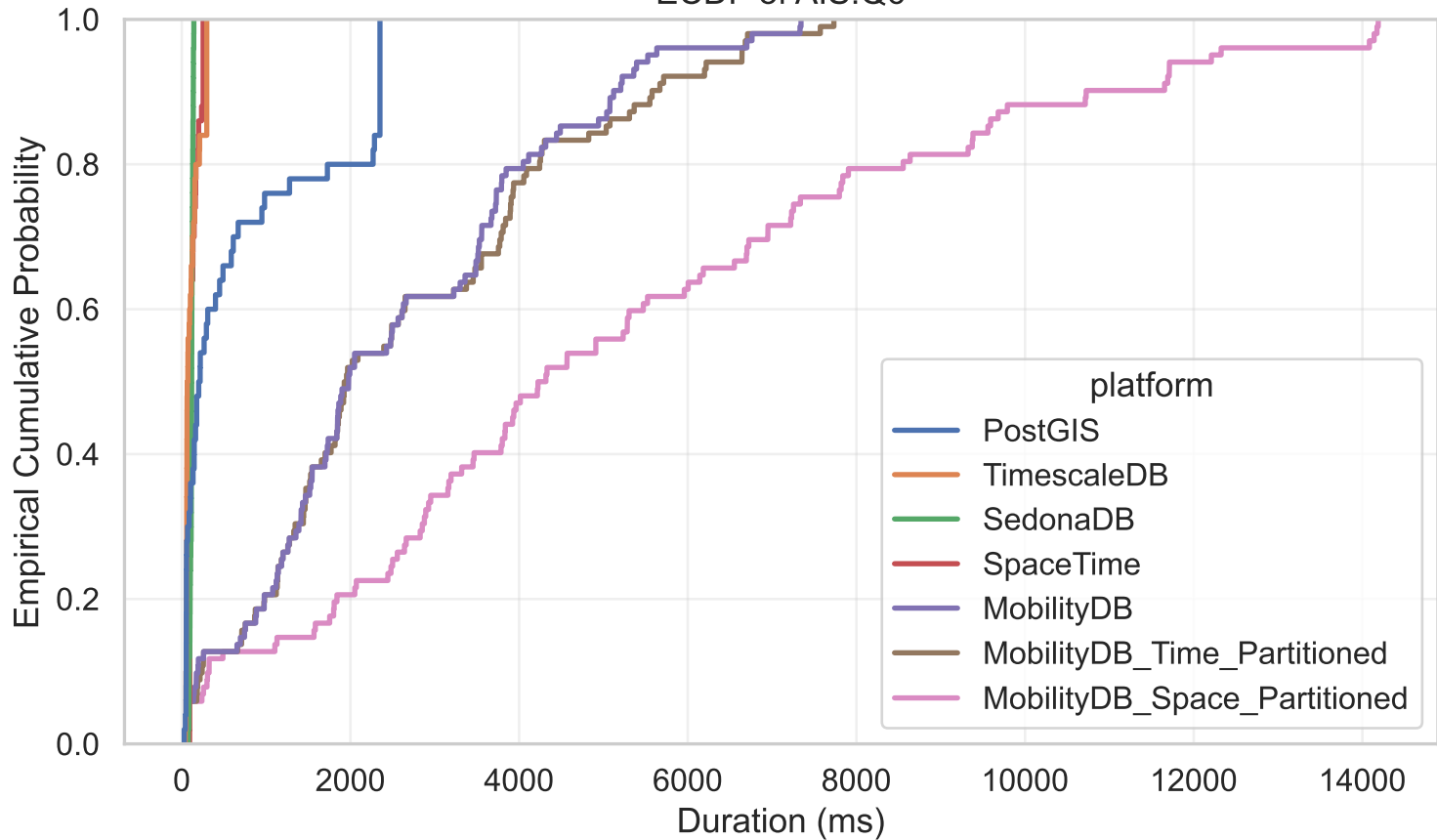
ECDF of AIS.Q6
