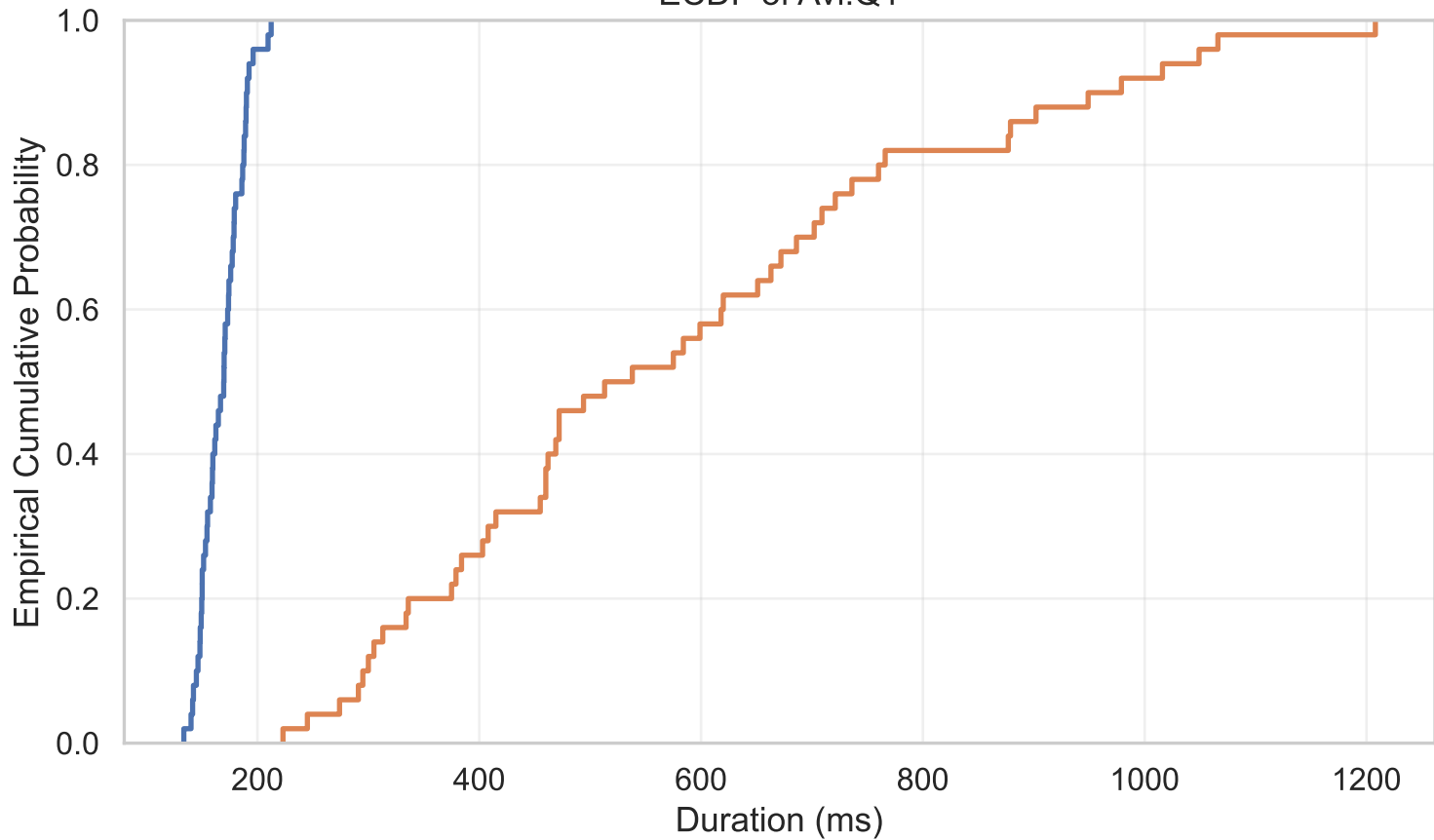
ECDF of Avi.Q1
