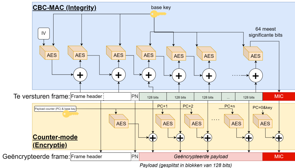
Figuur 5.24: CCMP: confidentiality en integrity in één.
