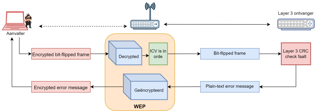
Figuur 5.17: Layer 3 misbruiken door corrupte, geblitflippte pakketjes, een gekende foutboodschap te laten genereren.
