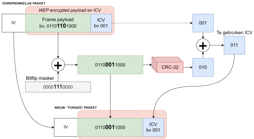
Figuur 5.16: De bitflip aanval.
