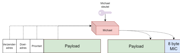
Figuur 5.21: Het aanmaken van een MIC met Michael.
