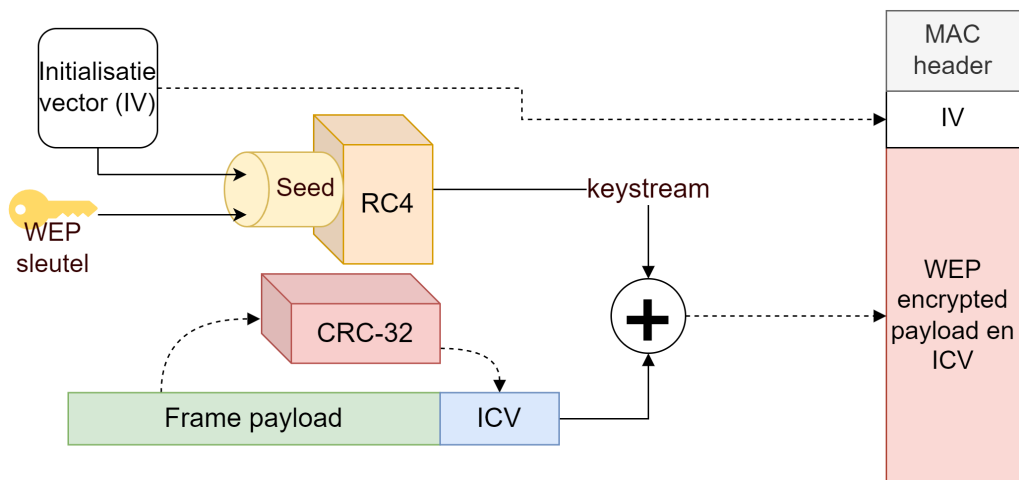
Figuur 5.12: WEP encryptie.
