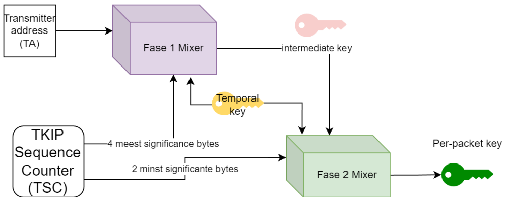
Figuur 5.22: Het mengen van de verschillende sleutels naar een sleutel die ieder pakketje verandert.
