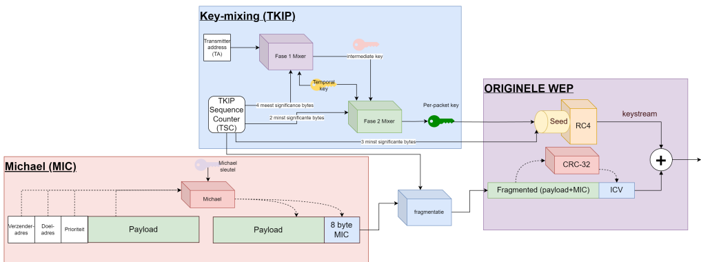
Figuur 5.23: WPA1 in volle glorie.
