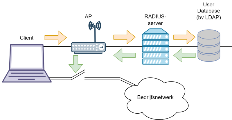
Figuur 5.18: Port-based authenticatie met 802.1X.
