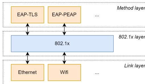
Figuur 5.19: De modulariteit van het 802.1X framework.
