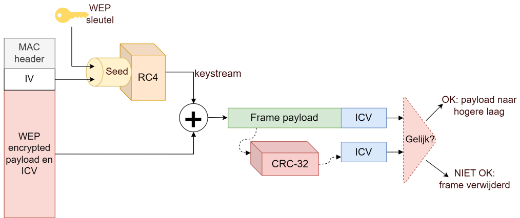
Figuur 5.13: WEP decryptie.
