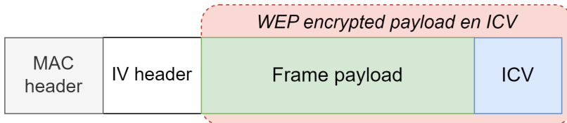
Figuur 5.11: WEP frame lay-out.
