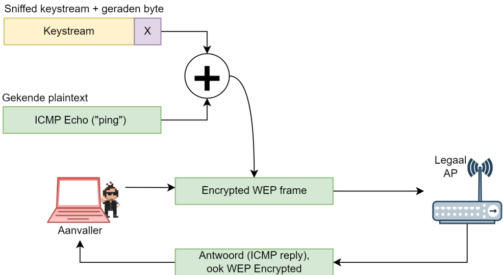
Figuur 5.15: Keystreams byte per byte groeien.
