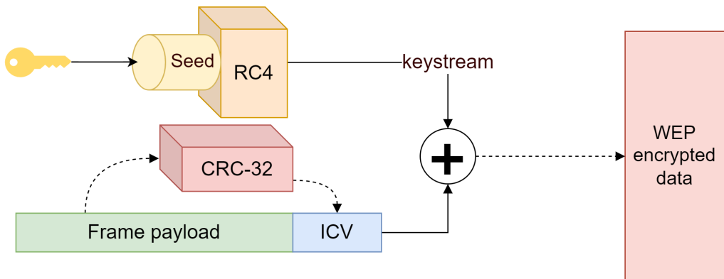
Figuur 5.9: Een vereenvoudigde voorstelling van WEP in z'n geheel.
