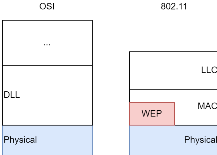
Figuur 5.8: De 802.11 stack (rechts) ten opzichte van de OSI stack.
