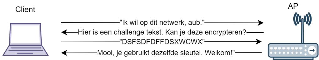
Figuur 5.7: De shared-key authentication aan de start van de verbinding.
