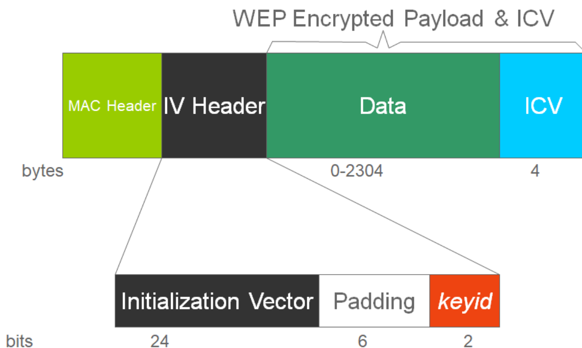
Figuur 0.4: WEAP frame layout
