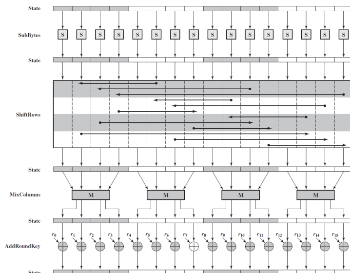
Figuur 0.13: AES encryptie (Bron wikipedia)
