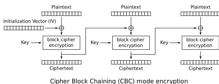
Figuur 0.12: CBC encryptie (Bron wikipedia)
