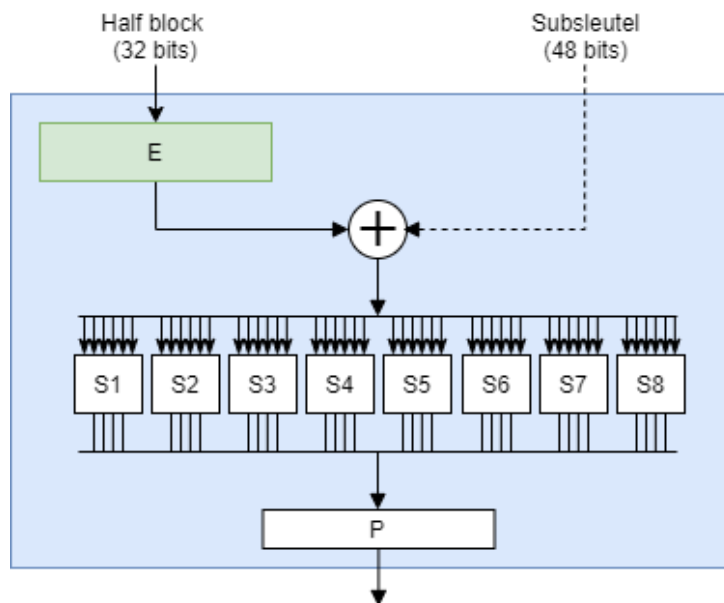
Figuur 0.9: Binnenin de F-operatie
