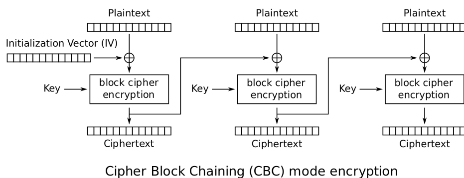
Figuur 0.15: CBC encryptie (Bron wikipedia)
