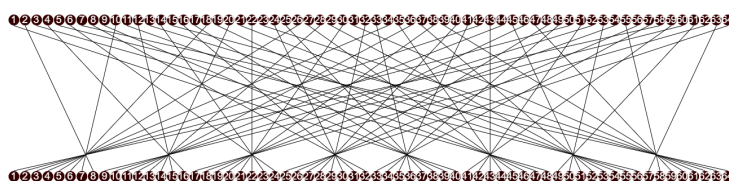
Figuur 0.8: De Initiële permutatie
