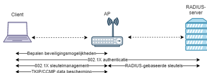
Figuur 0.19: Het authenticatie-proces op een wifi-netwerk met 802.1X (Enterprise-mode)
