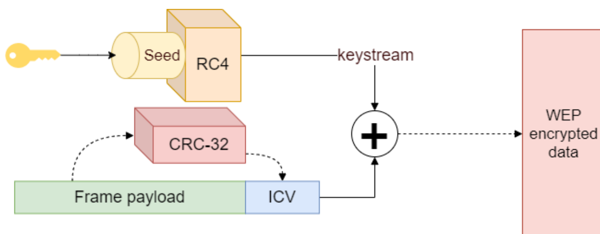
Figuur 0.8: WEP in z'n geheel
