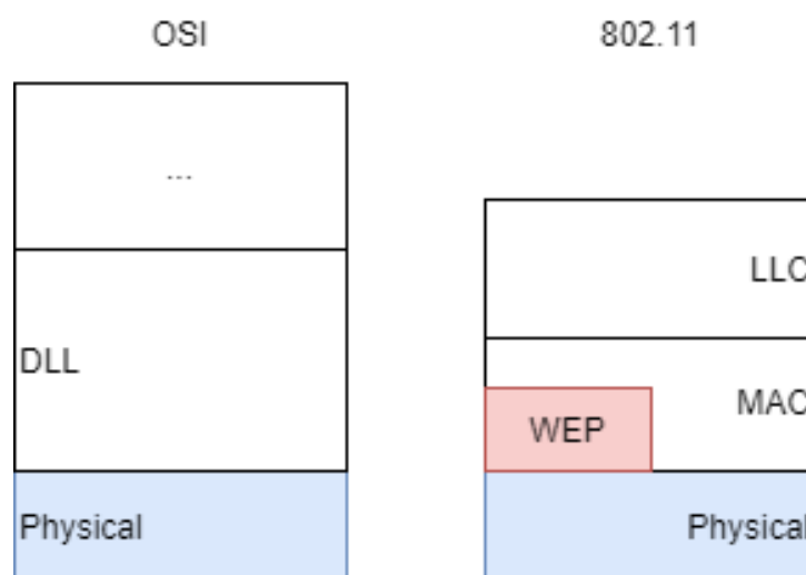
Figuur 0.7: De 802.11 stack (rechts) ten opzichte van de OSI stack
