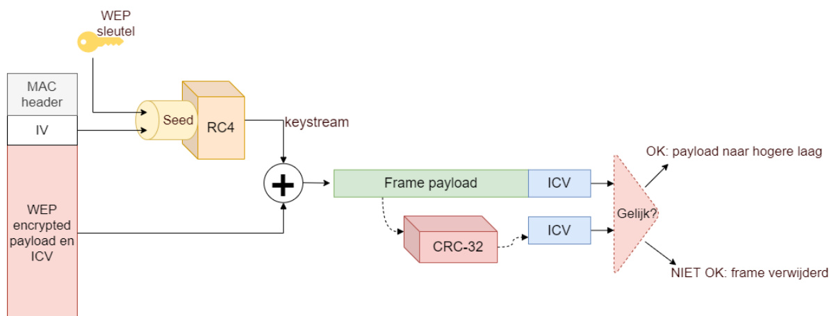
Figuur 0.12: WEP decryptie
