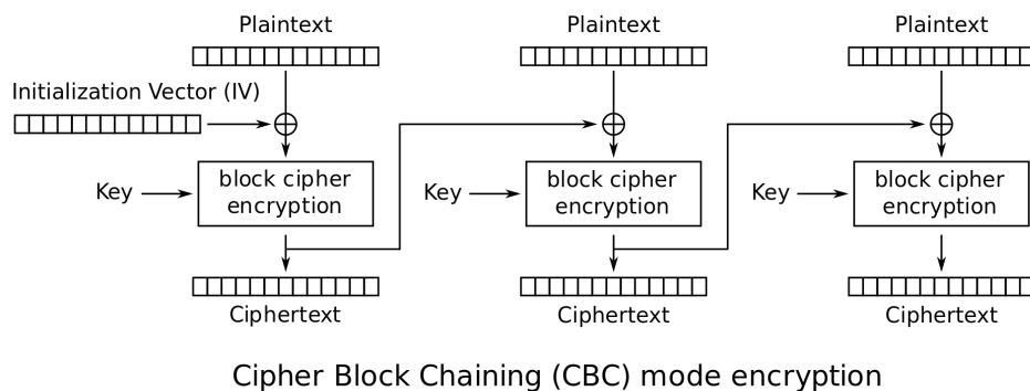
Figuur 4.18: CBC encryptie (Bron wikipedia).
