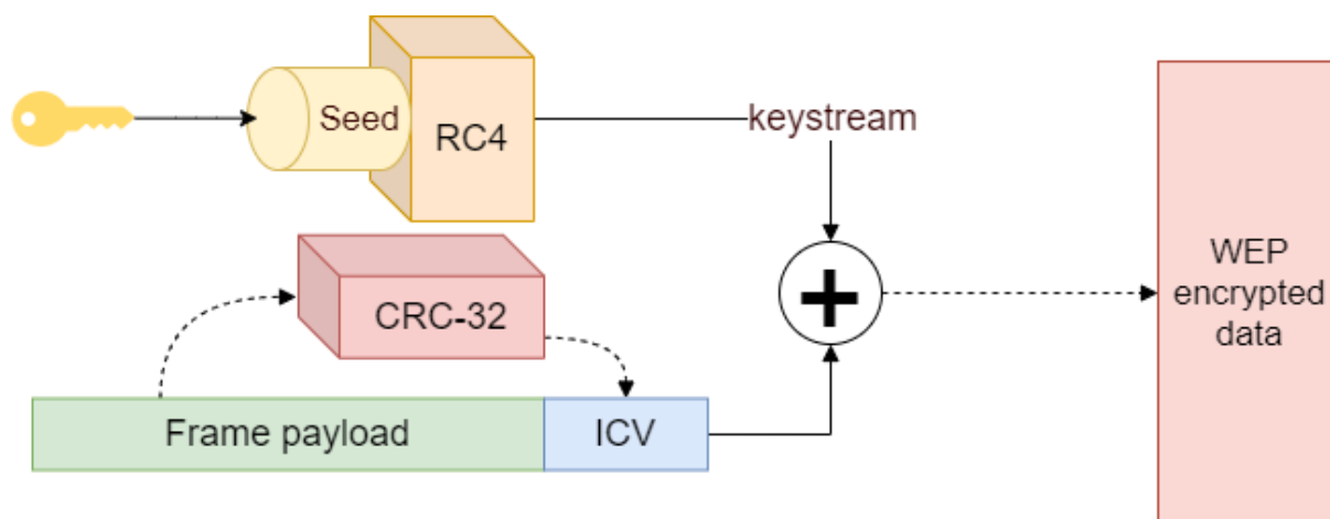
Figuur 8: WEP in z'n geheel
