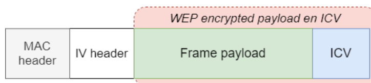
Figuur 10: WEP frame layout
