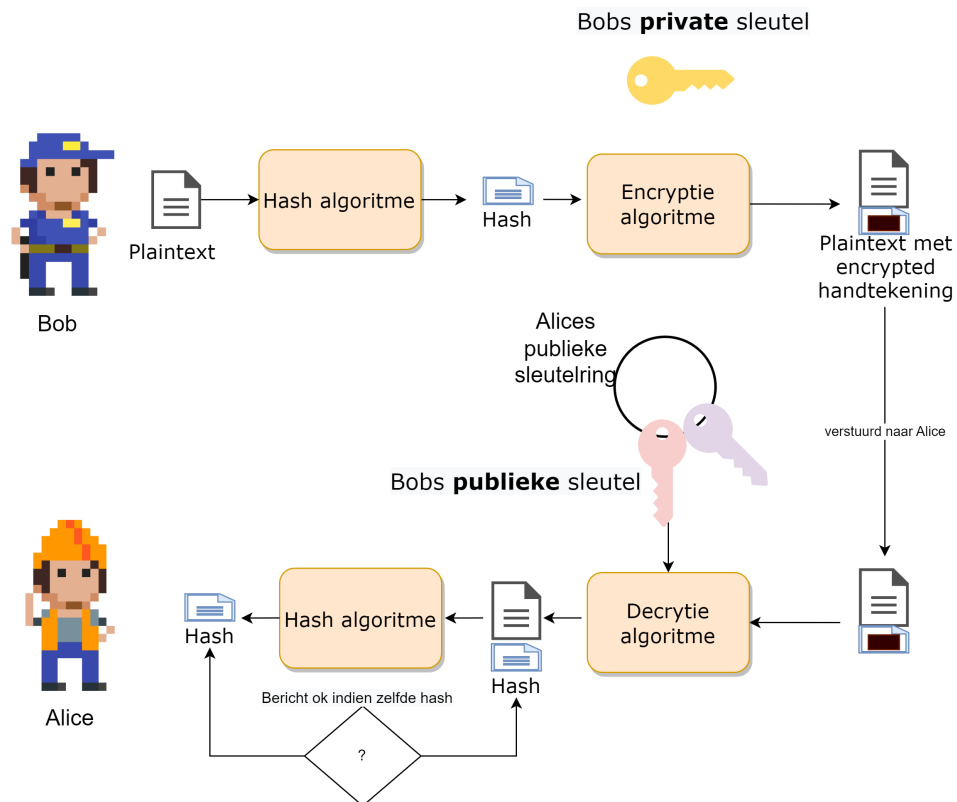
Figuur 4.26: Het volledig proces bij een digitale handtekening.
