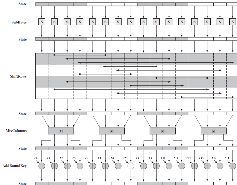
Figuur 4.20: AES encryptie (Bron wikipedia).
