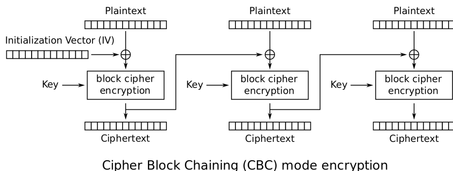
Figuur 4.19: CBC encryptie (Bron wikipedia).
