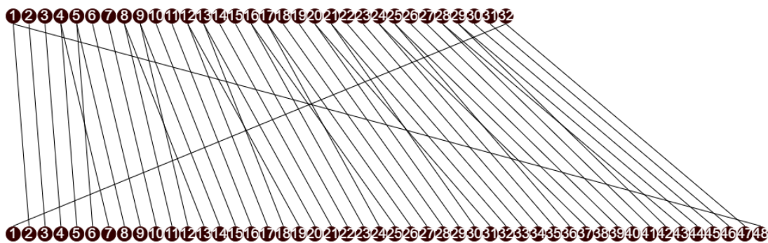
Figuur 4.14: De expansie van 32 naar 48 bits.
