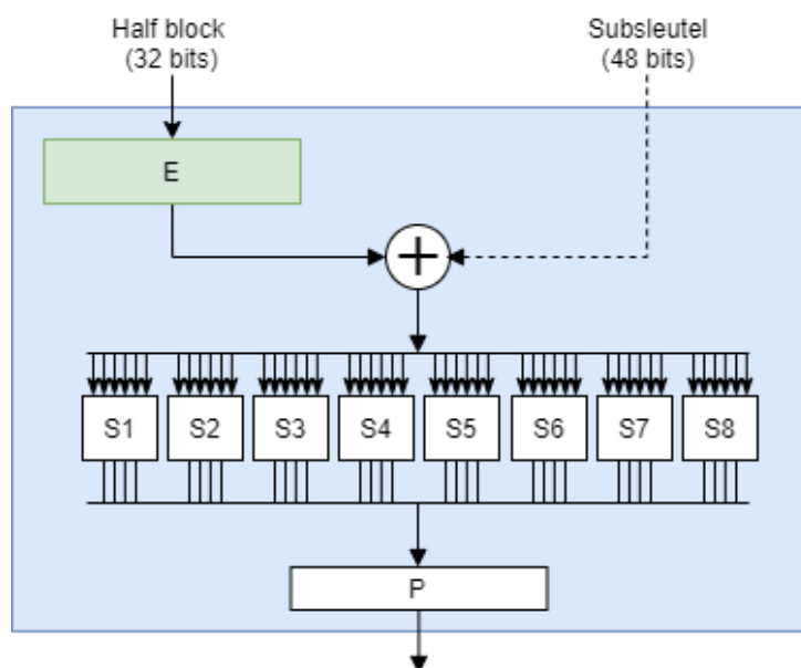
Figuur 5: Binnenin de F-operatie
