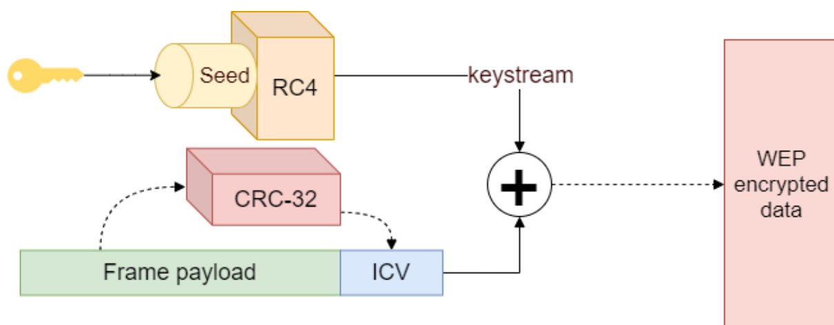
Figuur 2: WEP in z'n geheel
