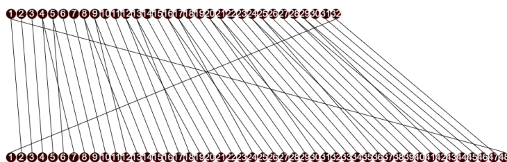
Figuur 6: De expansie van 32 naar 48 bits
