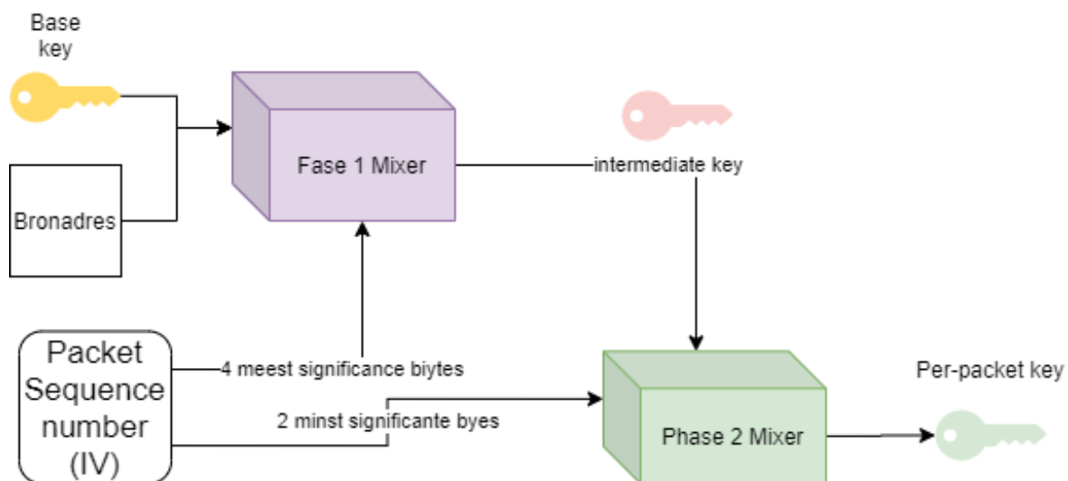
Figuur 21: Het mengen van de verschillende sleutels naar een sleutel die ieder pakketje verandert
