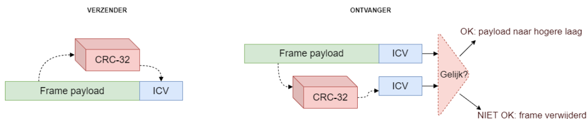
Figuur 9: Integrity check
