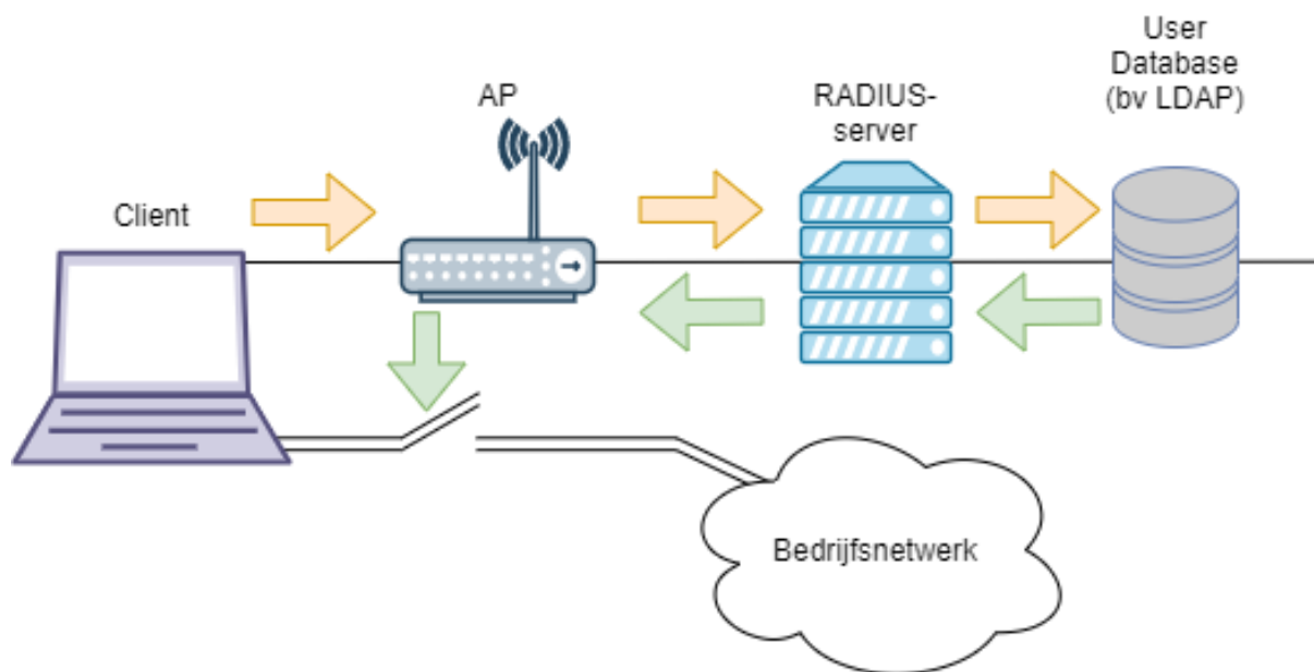
Figuur 17: Port-based authenticatie met 802.1X
