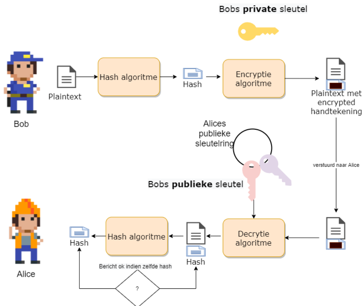
Figuur 22: Het volledig proces bij een digitale handtekening
