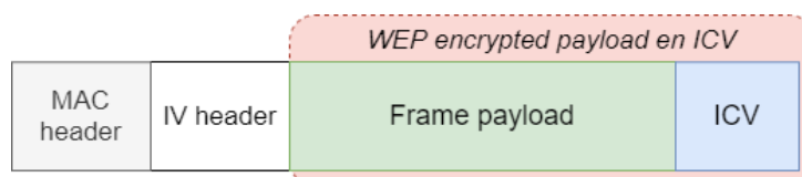
Figuur 10: WEP frame layout
