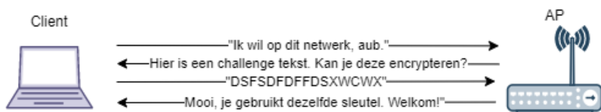
Figuur 6: De shared-key authentication aan de start van de verbinding
