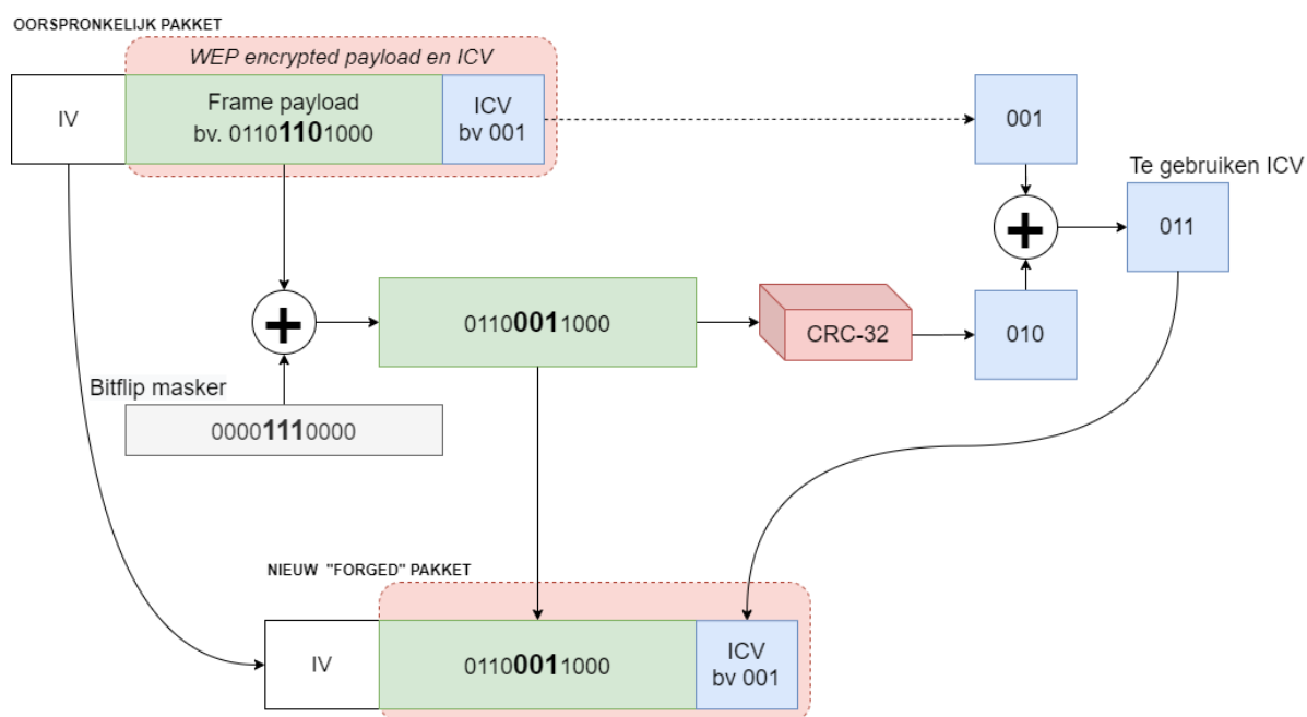
Figuur 15: De bitflip aanval
