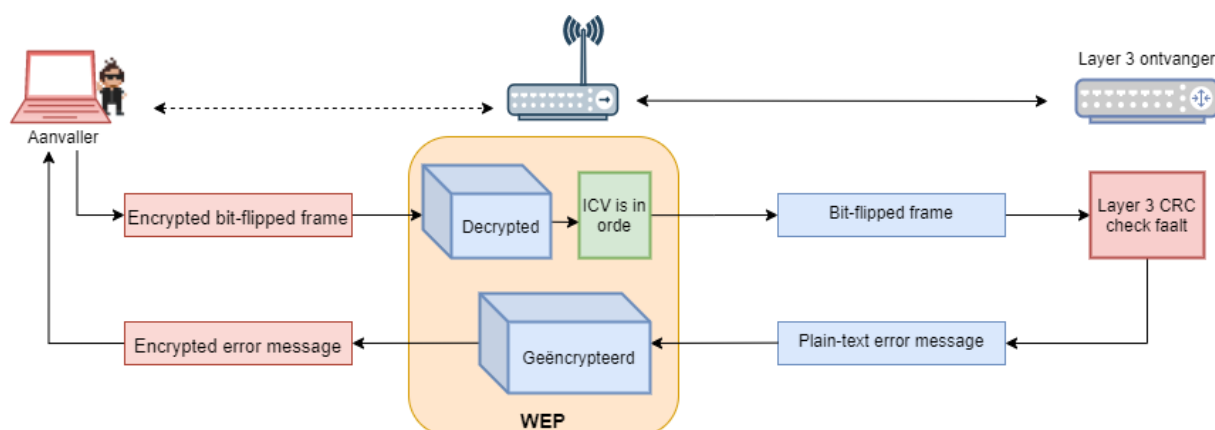
Figuur 16: Layer 3 misbruiken door corrupte, geblitflipte pakketjes, een gekende foutboodschap te laten genereren
