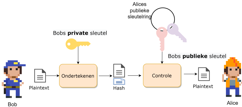
Figuur 4.24: Boodschappen ondertekenen met je private sleutel.
