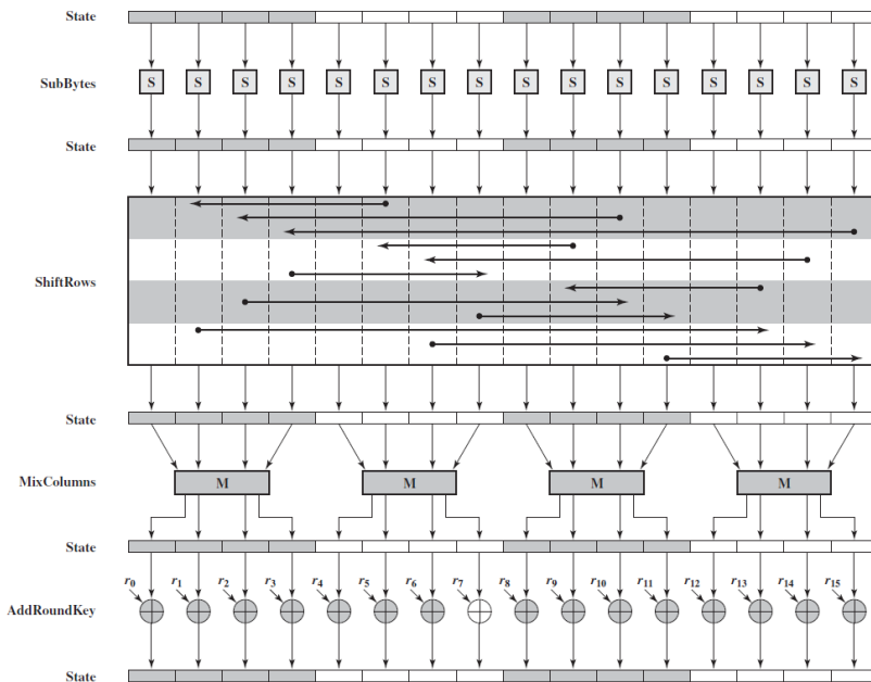
Figuur 4.19: AES encryptie (Bron wikipedia).
