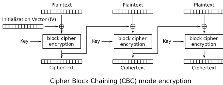
Figuur 4.18: CBC encryptie (Bron wikipedia).
