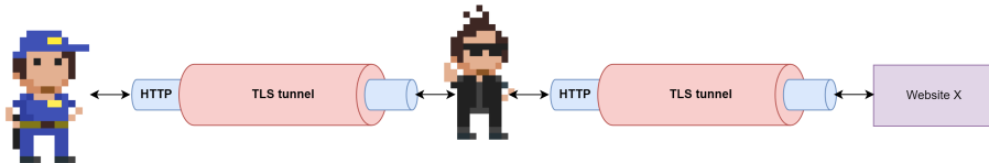
Figuur 4.36: Een man-in-the-middle aanval met TLS.
