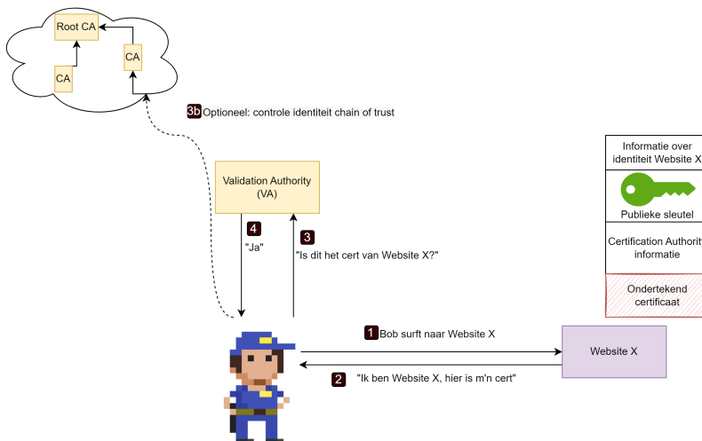
Figuur 4.29: Het certificaat tijdens het surfen.
