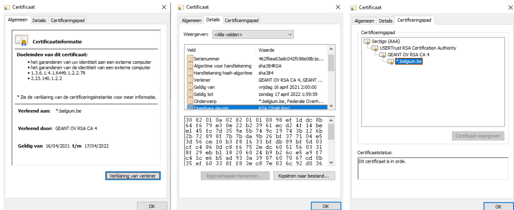
Figuur 4.31: Het certificaat van België.
