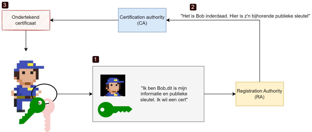
Figuur 4.27: Een certificaat registreren.
