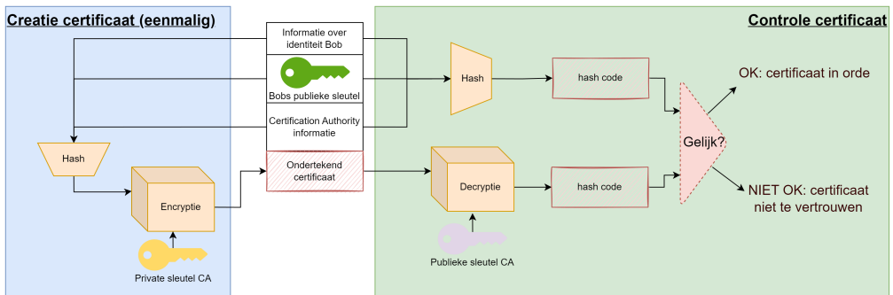
Figuur 4.28: Een certificaat aanmaken.
