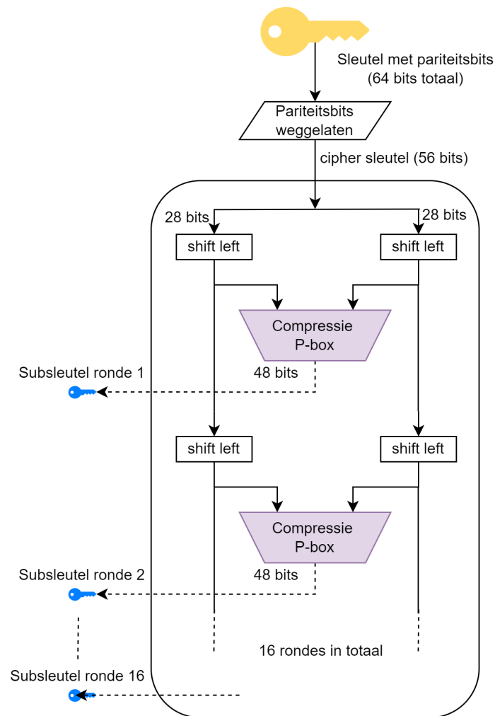
Figuur 4.15: De 16 rondes die telkens 1 subkey maken.
