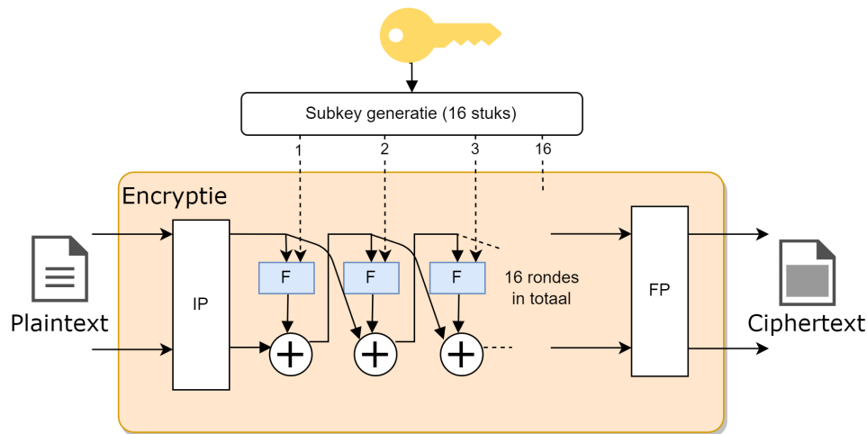
Figuur 4.10: DES encryptie. 16 Feistel-structuren na elkaar.
