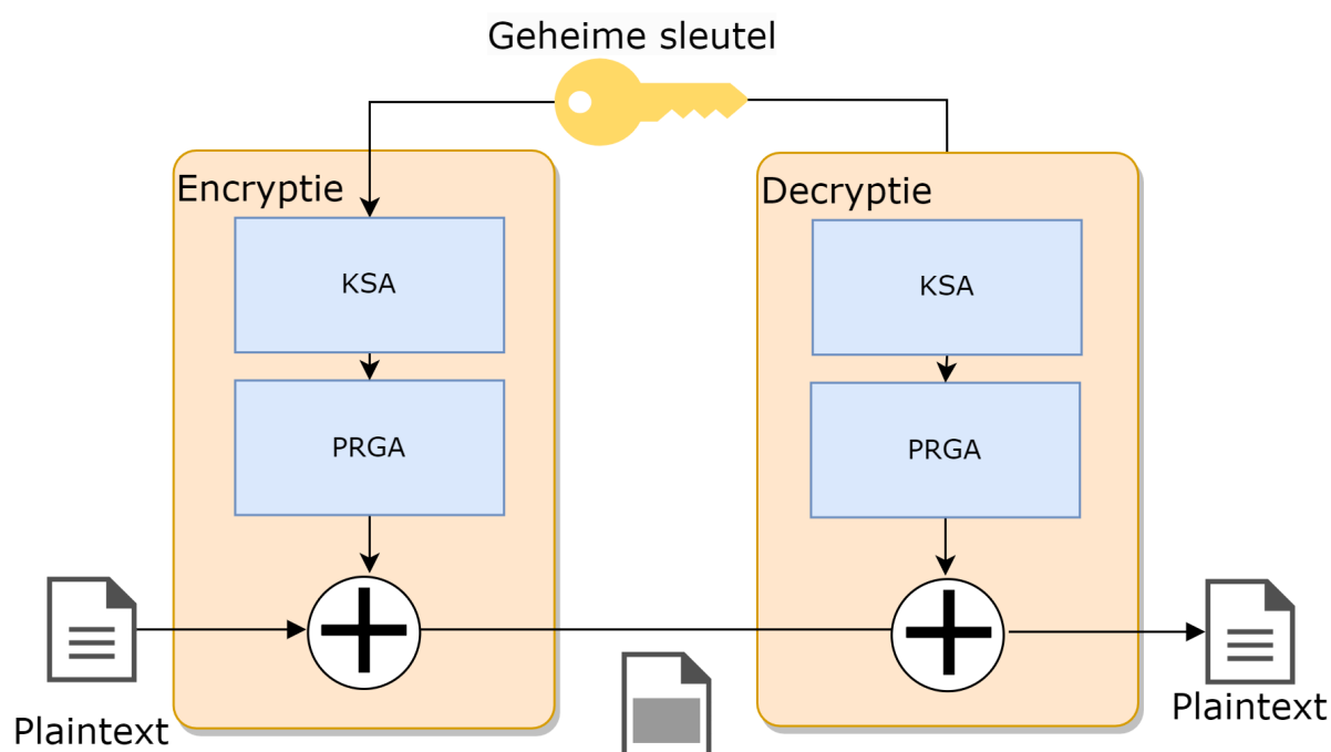
Figuur 4.8: RC4 tot op het bot.
