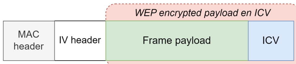
Figuur 5.10: WEP frame lay-out.
