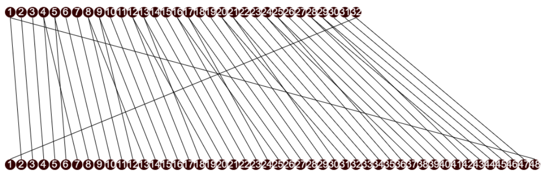
Figuur 4.13: De expansie van 32 naar 48 bits.
