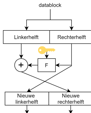
Figuur 4.9: Een enkele Feistel-structuur.
