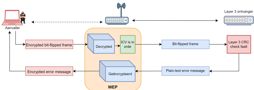
Figuur 5.17: Layer 3 misbruiken door corrupte, geblitflipte pakketjes, een gekende foutboodschap te laten genereren.
