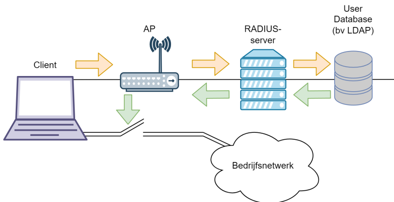
Figuur 5.18: Port-based authenticatie met 802.1X.
