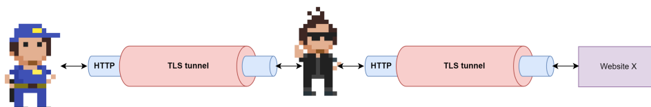
Figuur 4.33: Een man-in-the-middle aanval met TLS
