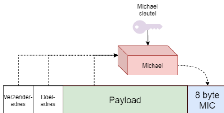
Figuur 5.20: Het aanmaken van een MIC met Michael
