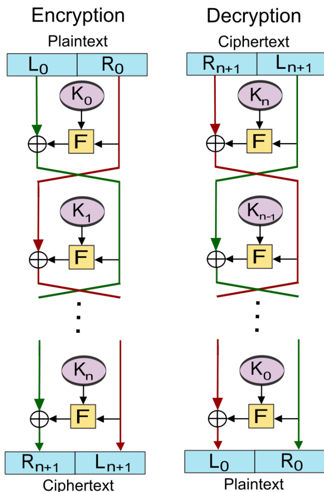
Figuur 4.9: Een reeks feistelstructuren na elkaar die in n rondes een plaintext encrypteren naar een ciphertext. Bron wikipedia
