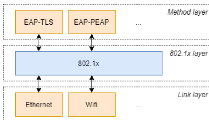
Figuur 5.18: De modulariteit van het 802.1X framework
