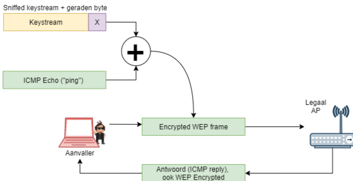
Figuur 5.14: Keystreams byte per byte groeien
