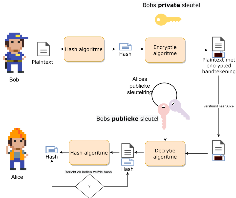
Figuur 4.25: Het volledig proces bij een digitale handtekening
