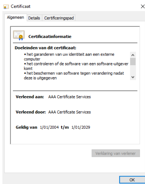
Figuur 4.32: Sectigo heeft een self-signed certificaat wat je herkent aan het feit dat de velden Verleend aan en Verleend door dezelfde waarde hebben.
