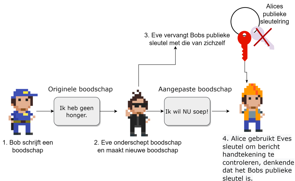
Figuur 4.26: Eve misbruikt het vertrouwen dat zit ingebouwd in het digitale handtekening proces
