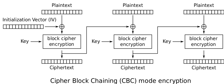
Figuur 4.18: CBC encryptie (Bron wikipedia)
