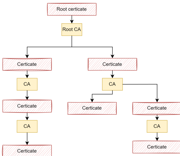
Figuur 4.30: De chain-of-trust: oh zo belangrijk bij digitale certificaten
