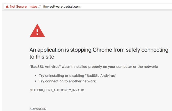
Figuur 4.36: De waarschuwing die Chrome genereert wanneer het een, potentiële, mitm-aanval detecteert
