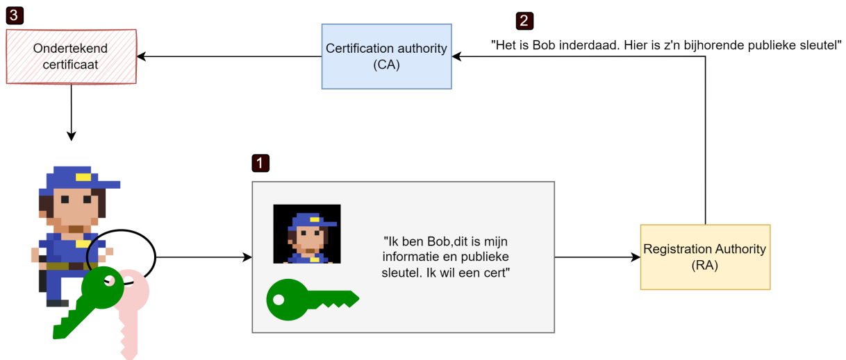
Figuur 4.27: Een certificaat registreren
