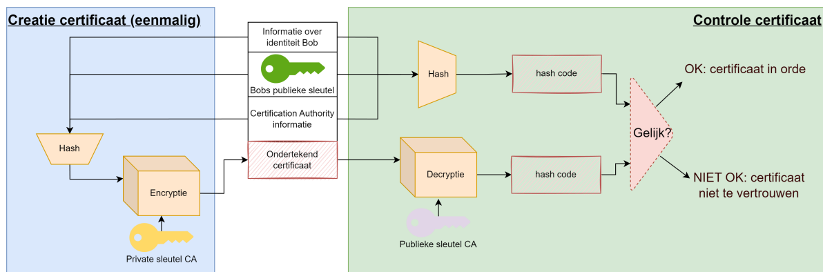
Figuur 4.28: Een certificaat aanmaken.
