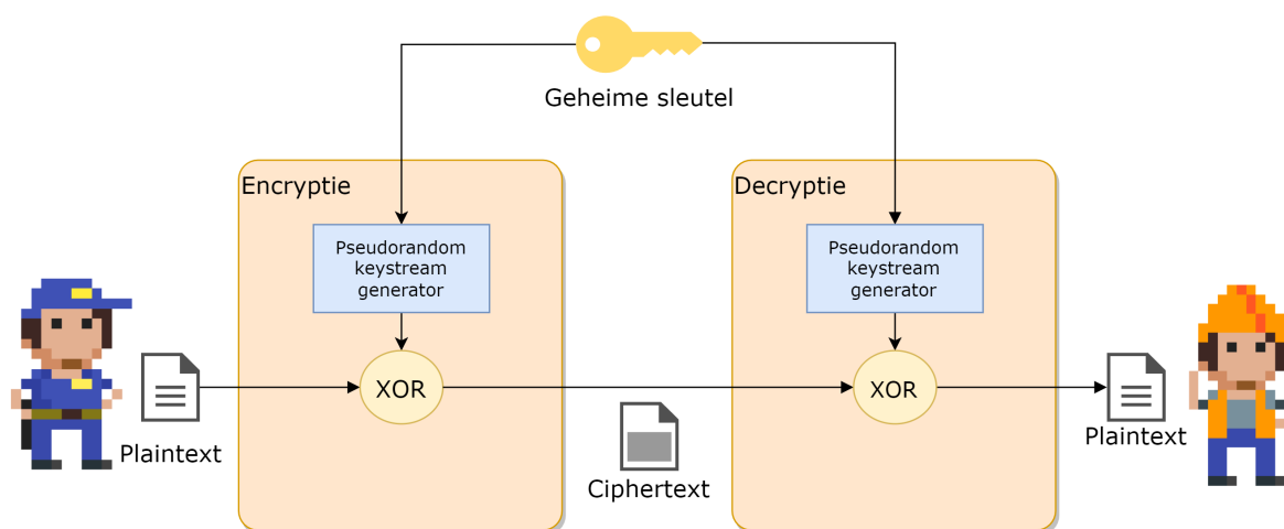
Figuur 4.7: Het streamcipher proces
