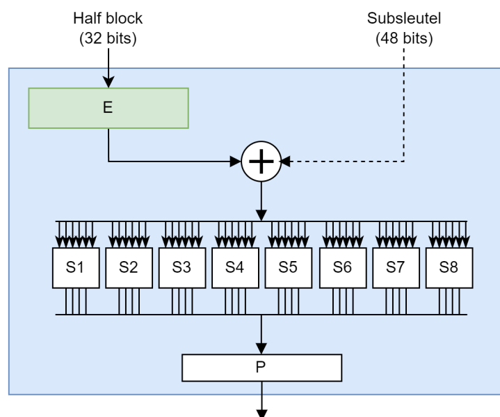
Figuur 4.12: Binnenin de F-operatie
