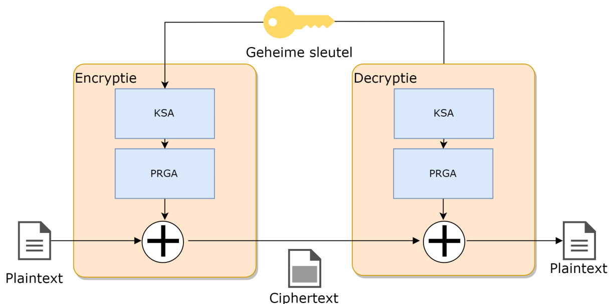
Figuur 4.8: RC4 tot op het bot
