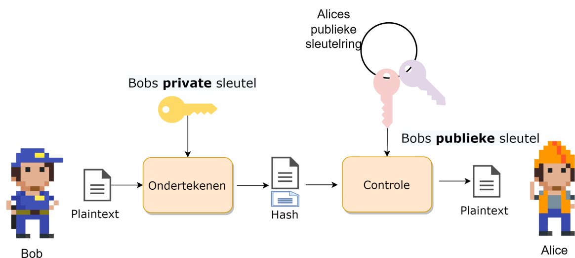
Figuur 4.24: Boodschappen ondertekenen met je private sleutel
