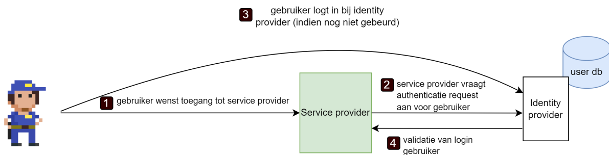
Figuur 6.9: Een vereenvoudigd single sign-on proces
