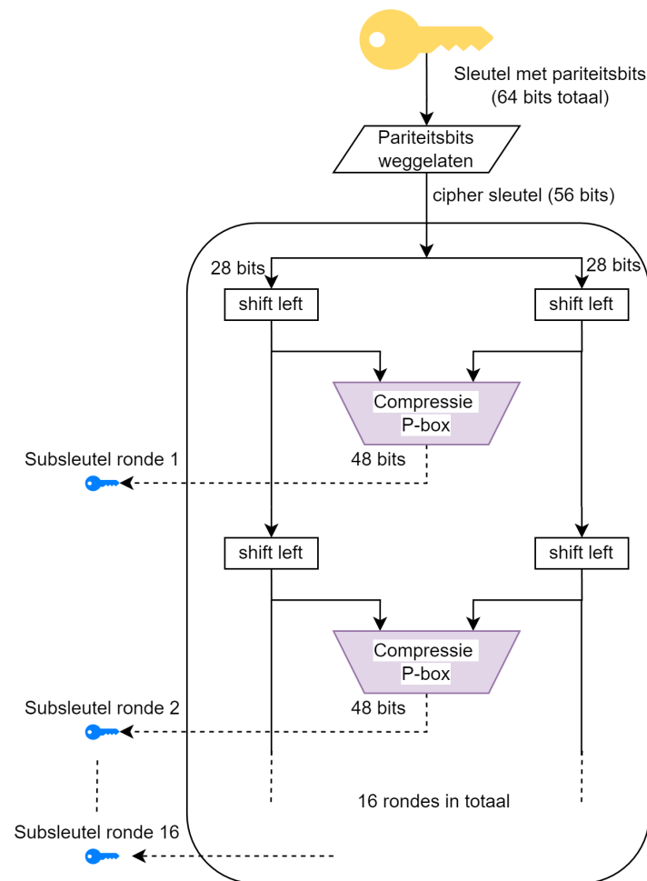
Figuur 4.15: De 16 rondes die telkens 1 subkey maken.
