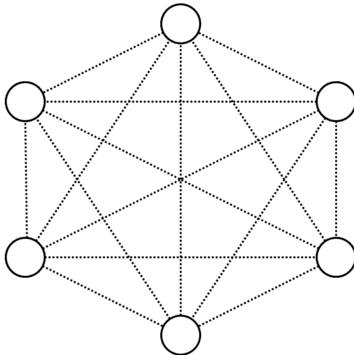
Figuur 4.20: Bij 6 gebruikers zijn er al 15 sleutels nodig.
