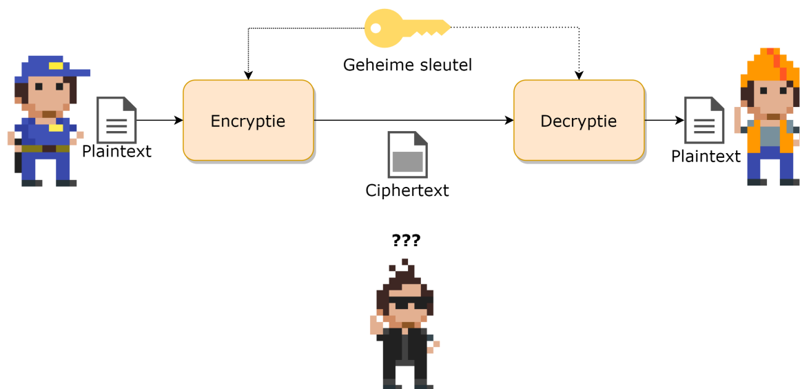
Figuur 4.6: Het basismodel van symmetrische encryptie
