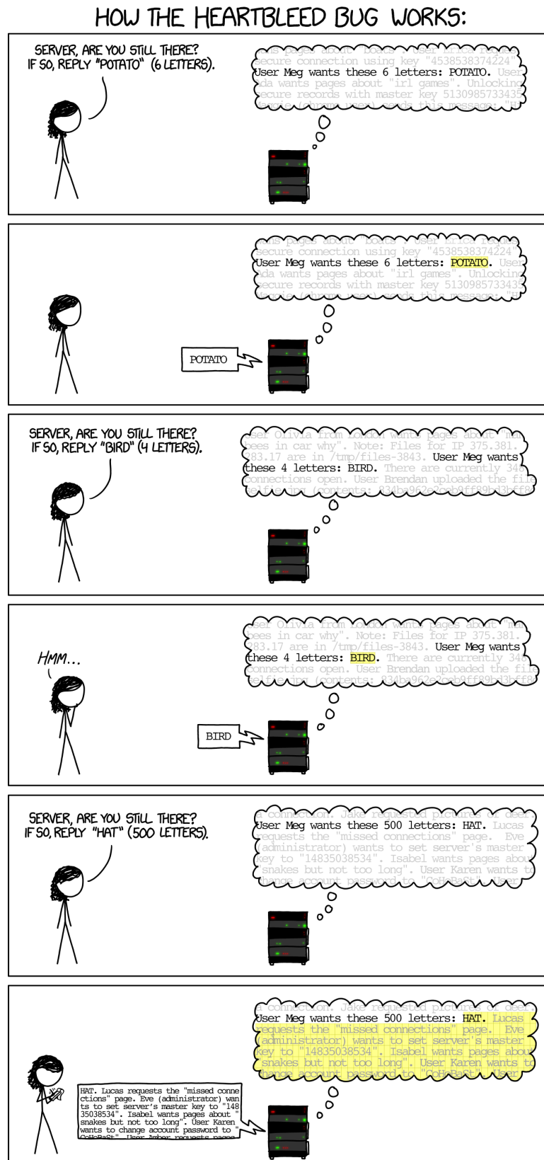
Figuur 3.18: De briljante xkcd.com heeft legt perfect uit hoe Heartbleed werkt
