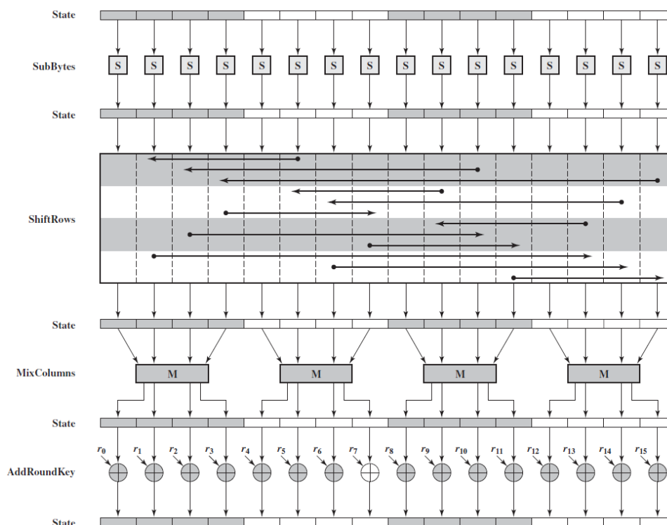
Figuur 4.19: AES encryptie. (Bron wikipedia)
