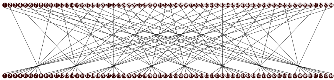
Figuur 4.11: De Initiële permutatie
