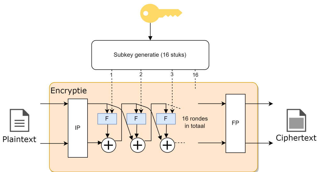
Figuur 4.10: DES encryptie. 16 feistel structuren na elkaar.
