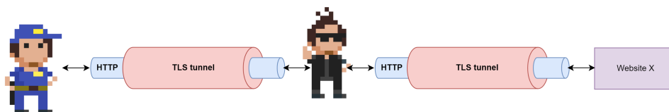
Figuur 4.35: Een man-in-the-middle aanval met TLS
