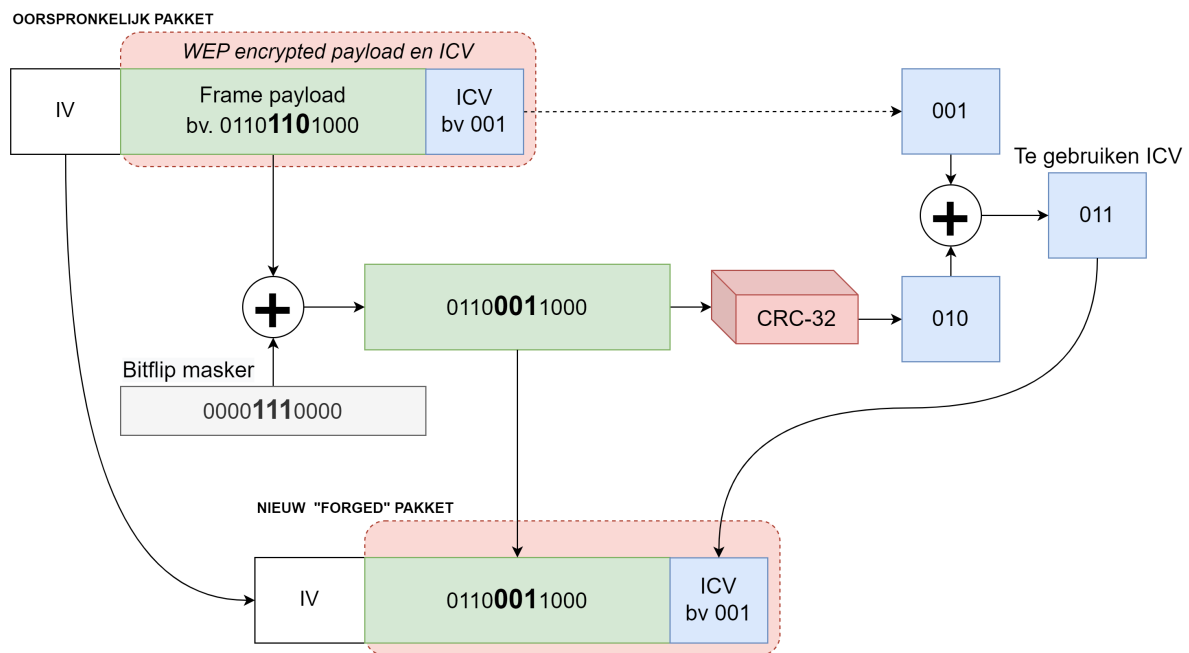
Figuur 5.15: De bitflip aanval
