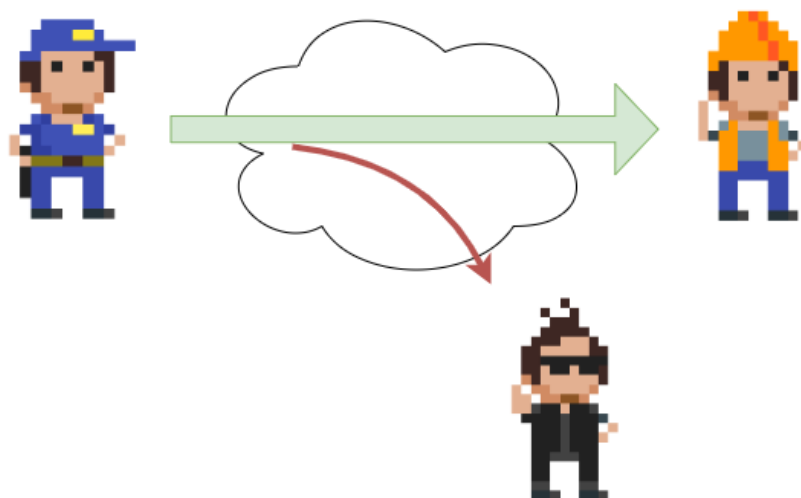
Figuur 3.6: Passieve aanval, type 1: sniffing
