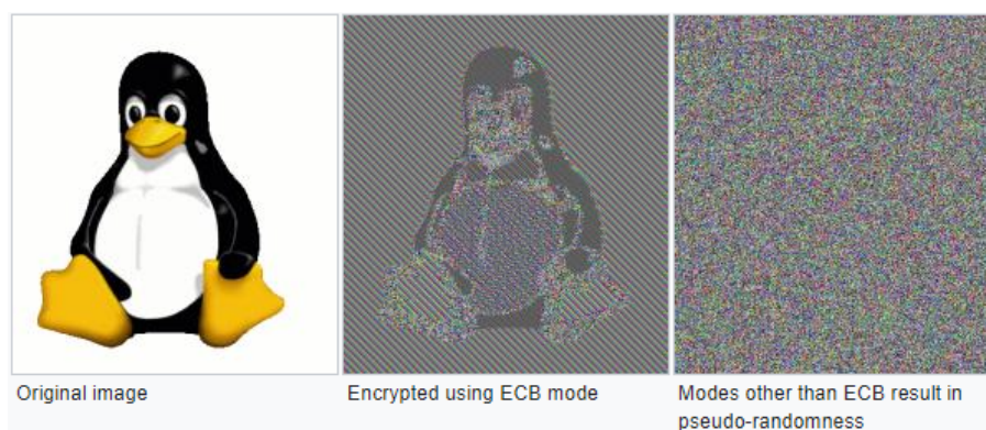
Figuur 4.17: Het volgend voorbeeld toont een (overdreven) manier waarom ECB minder veilig is dan de modes die we nog gaan behandelen (Bron wikipedia)
