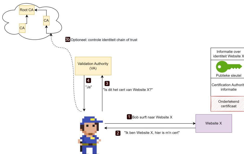
Figuur 4.29: Het certificaat tijdens het surfen.
