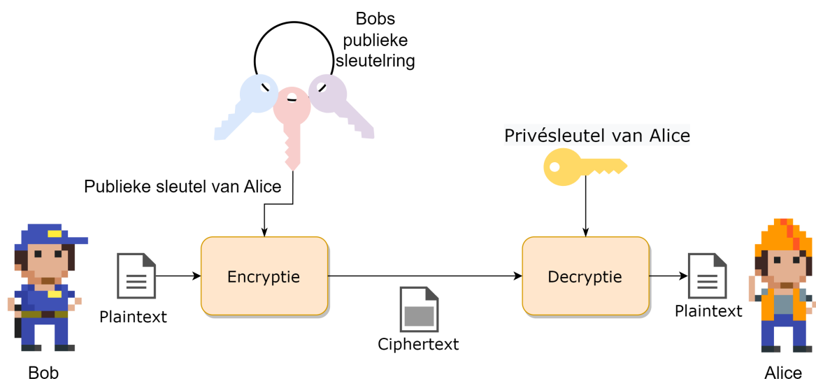
Figuur 4.21: Publieke crypto: Bob gebruikt de publieke sleutel van Alice om haar een beveiligd bericht te sturen.
