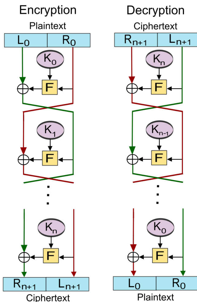
Figuur 9: Een reeks feistelstructuren na elkaar die in n rondes een plaintext encrypteren naar een ciphertext. Bron wikipedia
