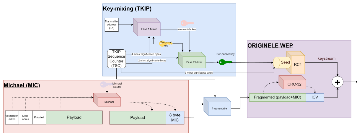
Figuur 5.22: WPA1 in volle glorie.
