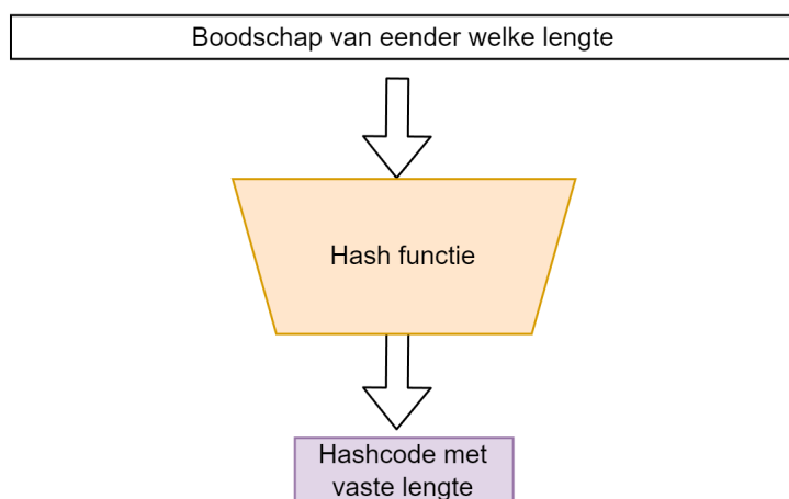
Figuur 4.24: Het hash proces.
