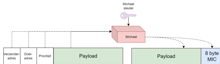
Figuur 5.20: Het aanmaken van een MIC met Michael.
