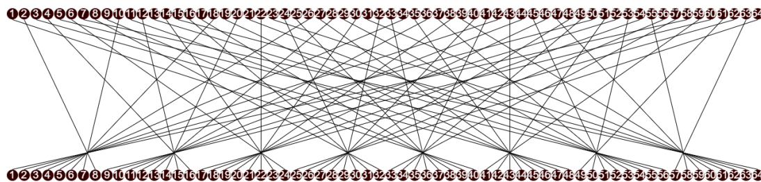
Figuur 4.11: De Initiële Permutatie.
