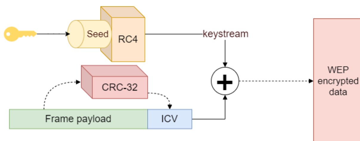
Figuur 2: WEP in z'n geheel
