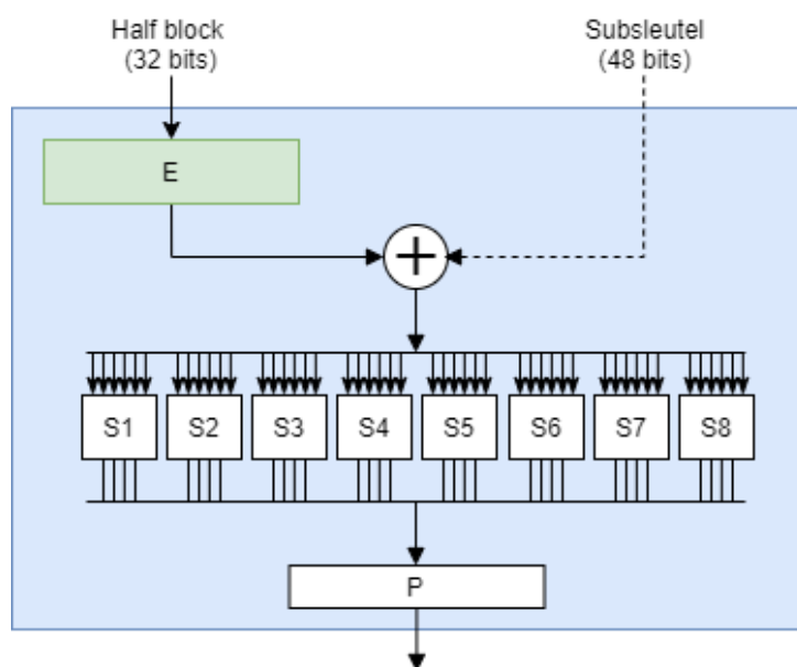
Figuur 5: Binnenin de F-operatie
