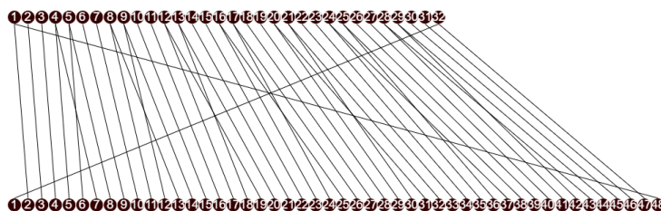
Figuur 6: De expansie van 32 naar 48 bits
