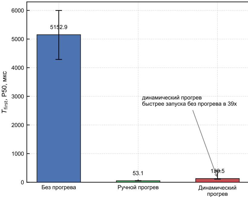
Задержка первого запроса после запуска
