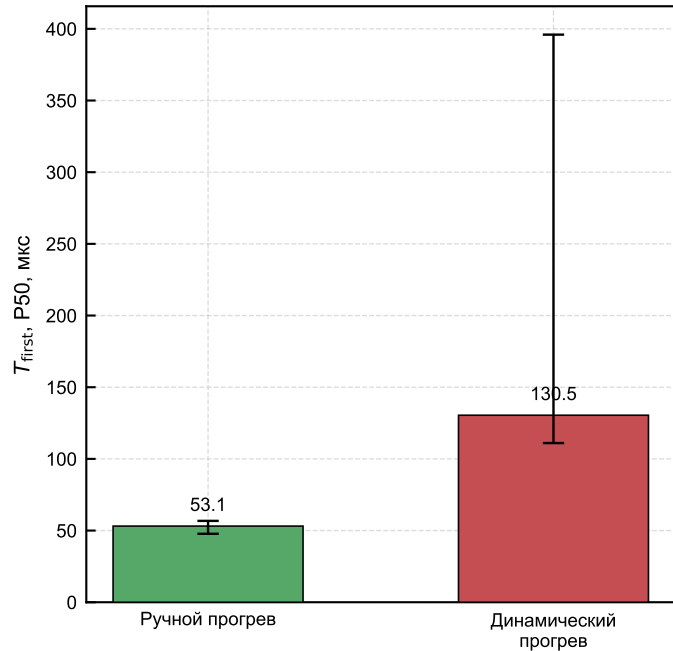
Сравнение прогретых сценариев
