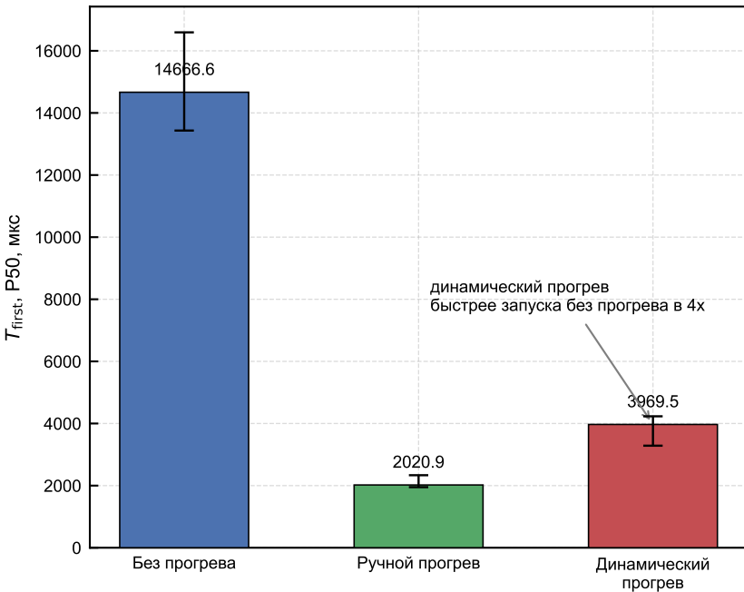
Задержка построения hashtable при первом запросе
