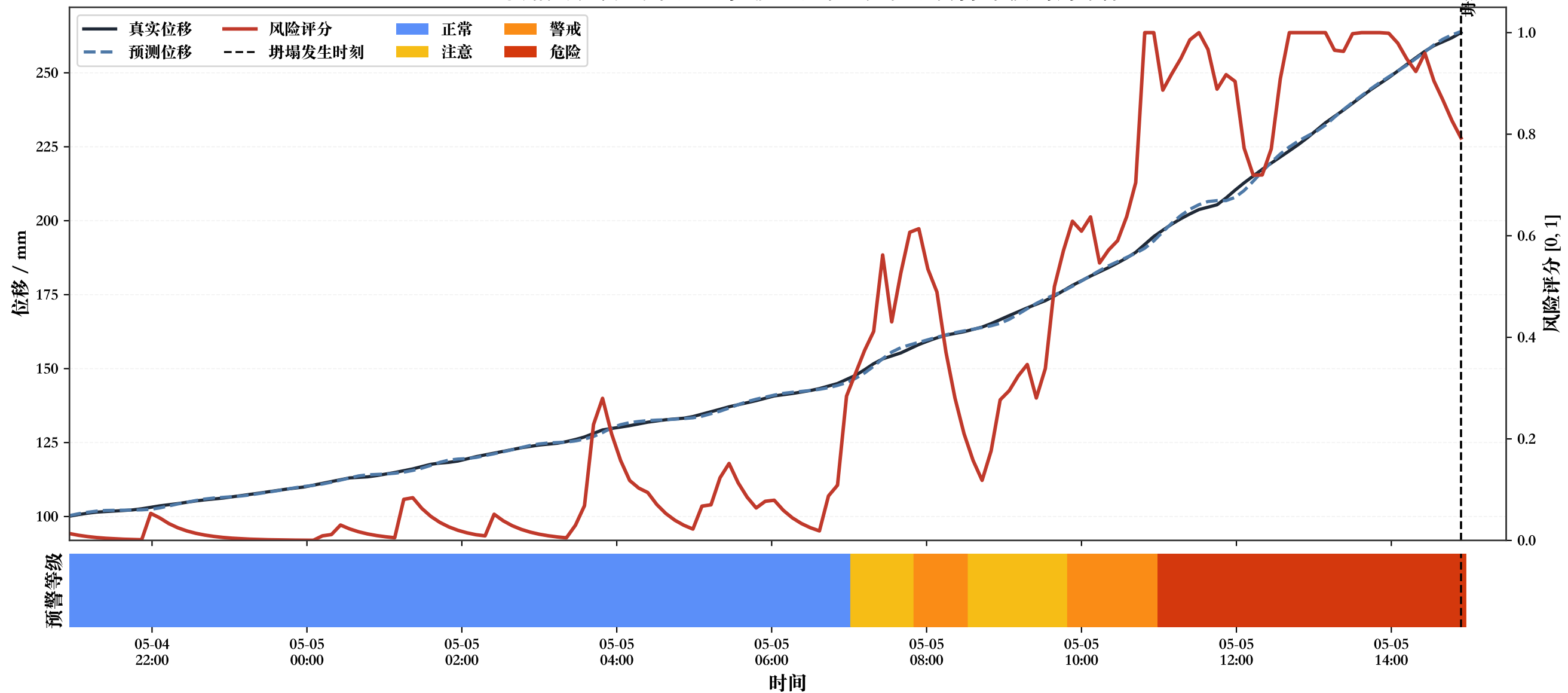
Dexing 露天矿坍塌案例的位移、风险评分与预警等级时序演化
