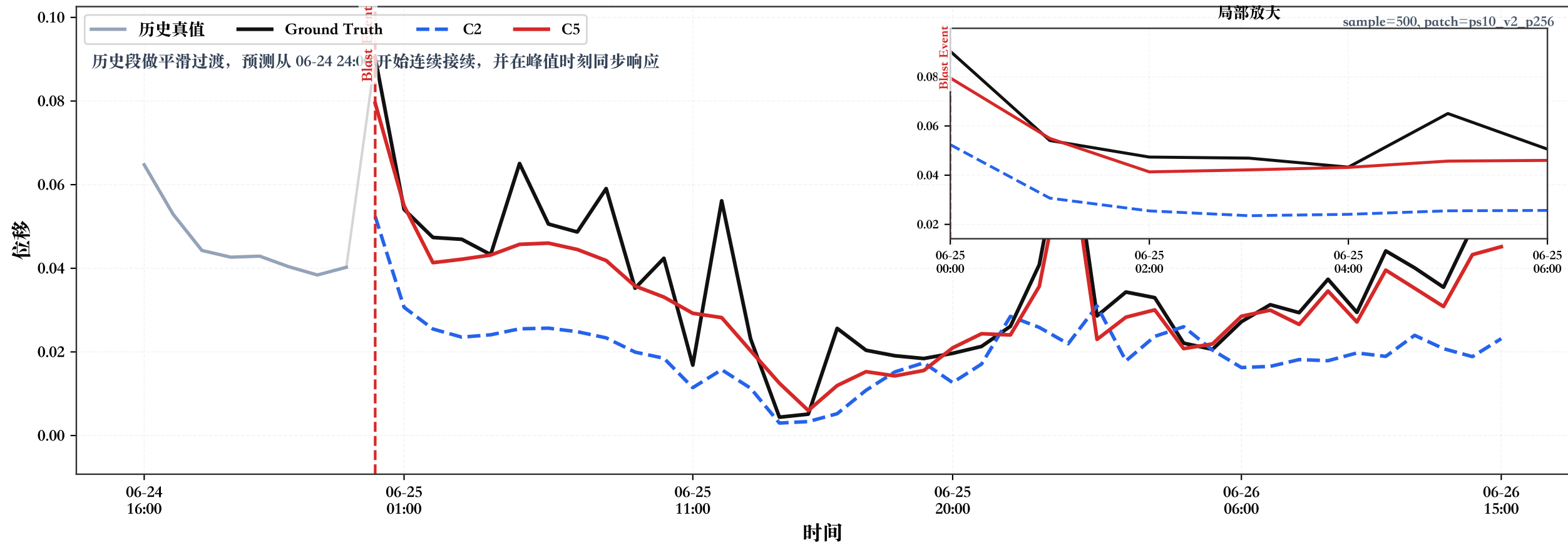
(b) 爆破冲击下的无延迟阶跃响应验证
