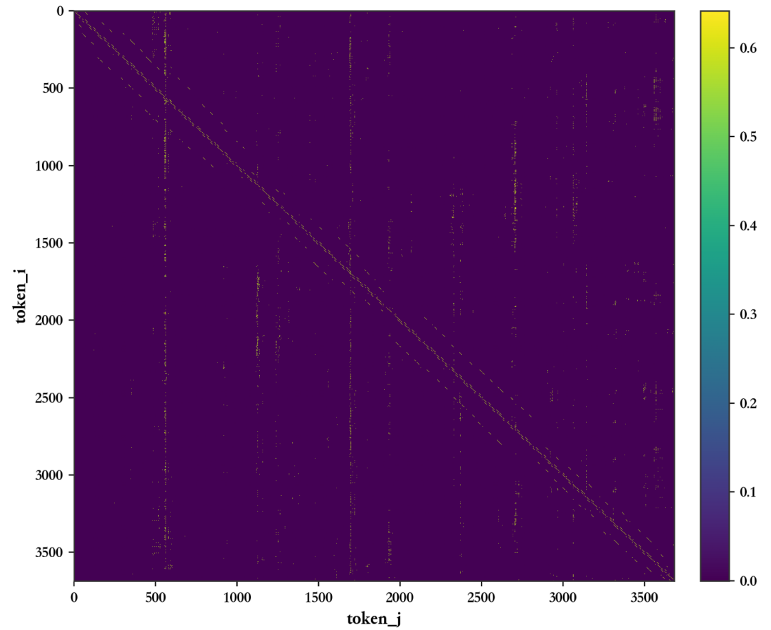
融合图
