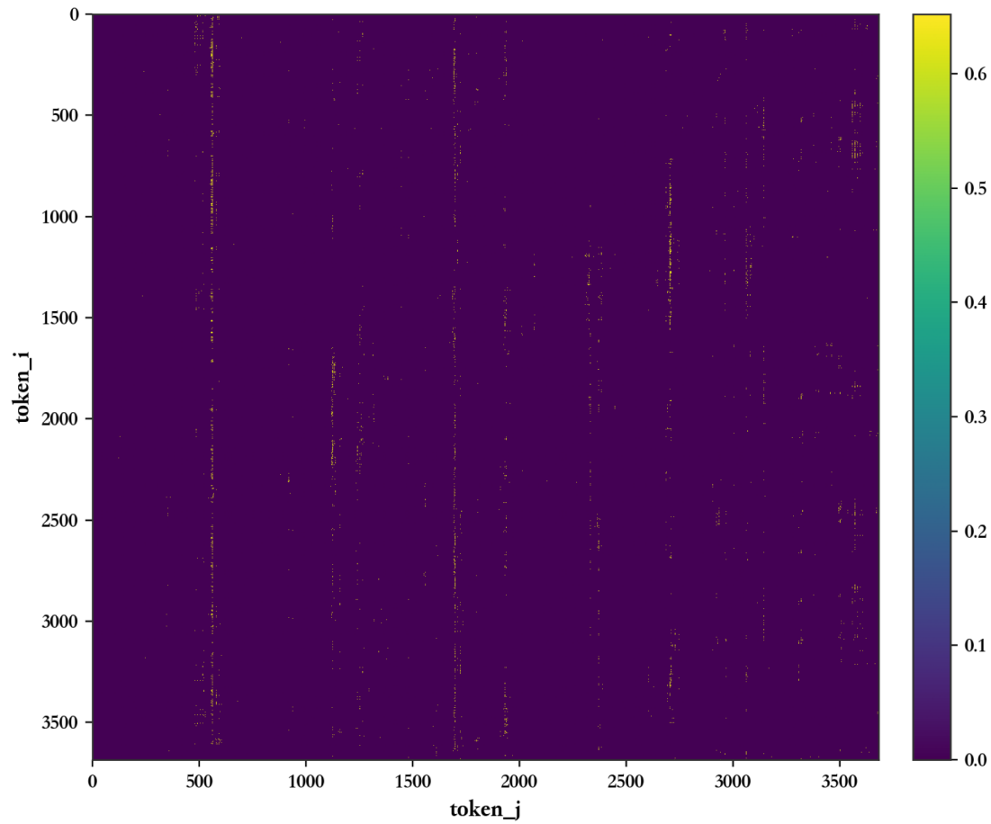
学习图
