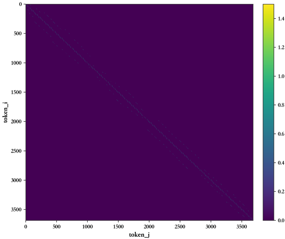
时空先验图
