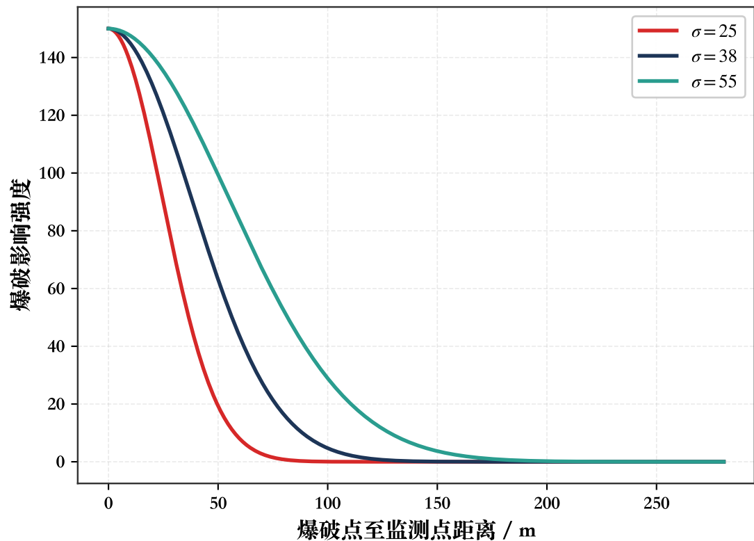
不同影响范围参数下的衰减对比
