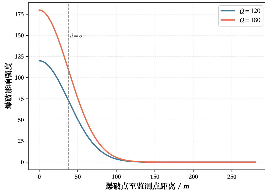
不同炸药量下的高斯衰减曲线
