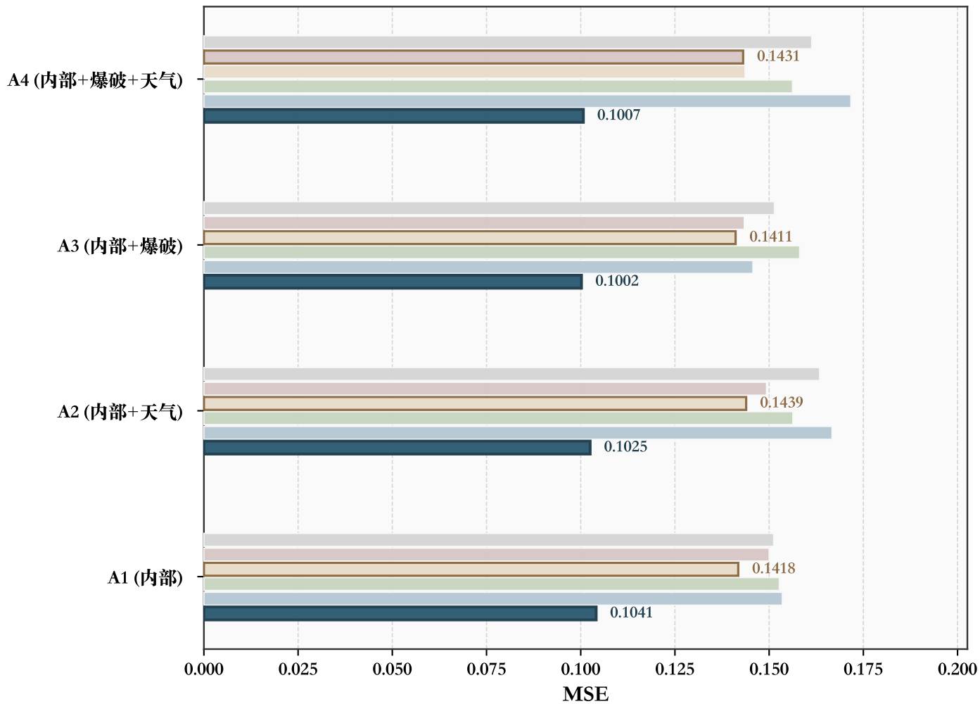
(a) MSE
