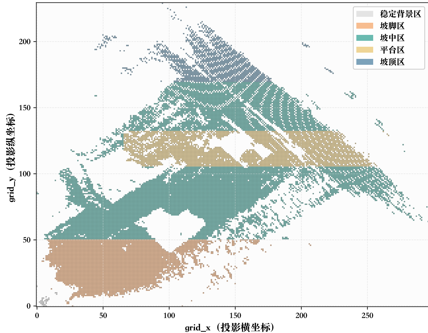
边坡工程分区示意图
