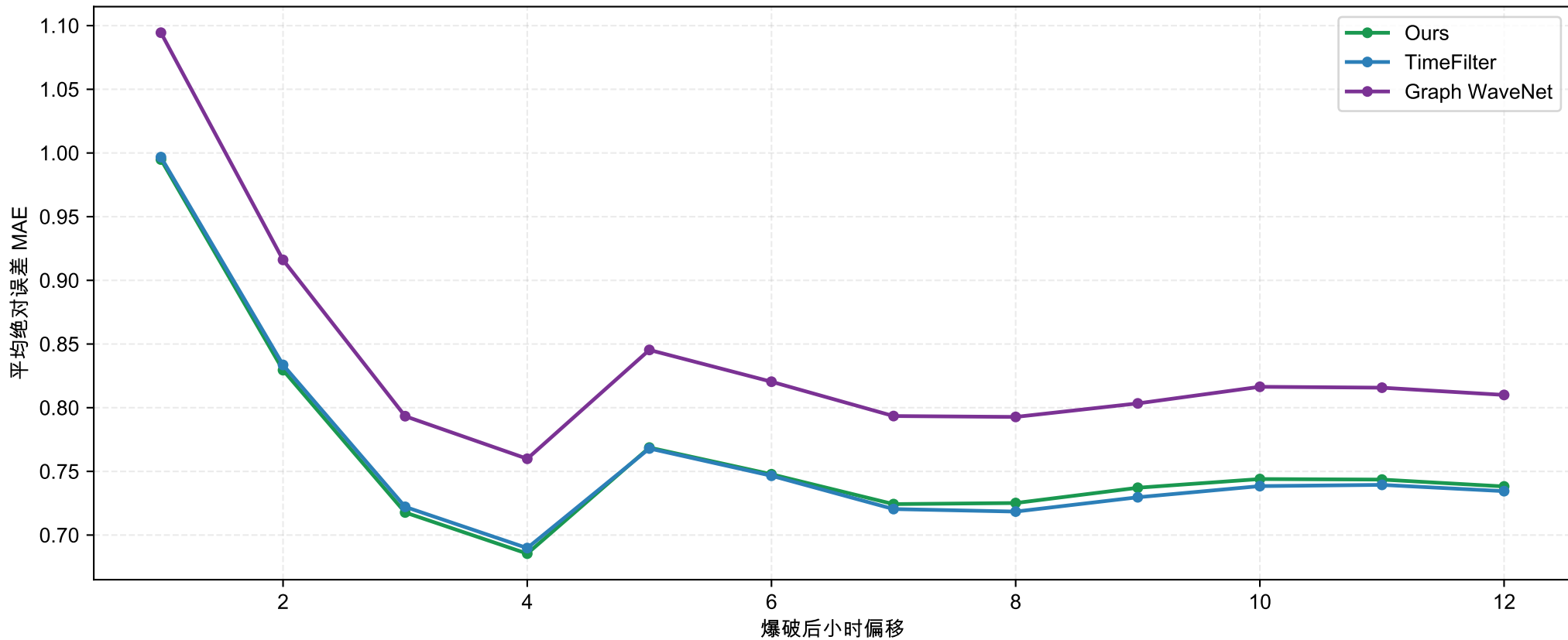
图3-4 爆破后误差随时间衰减曲线
