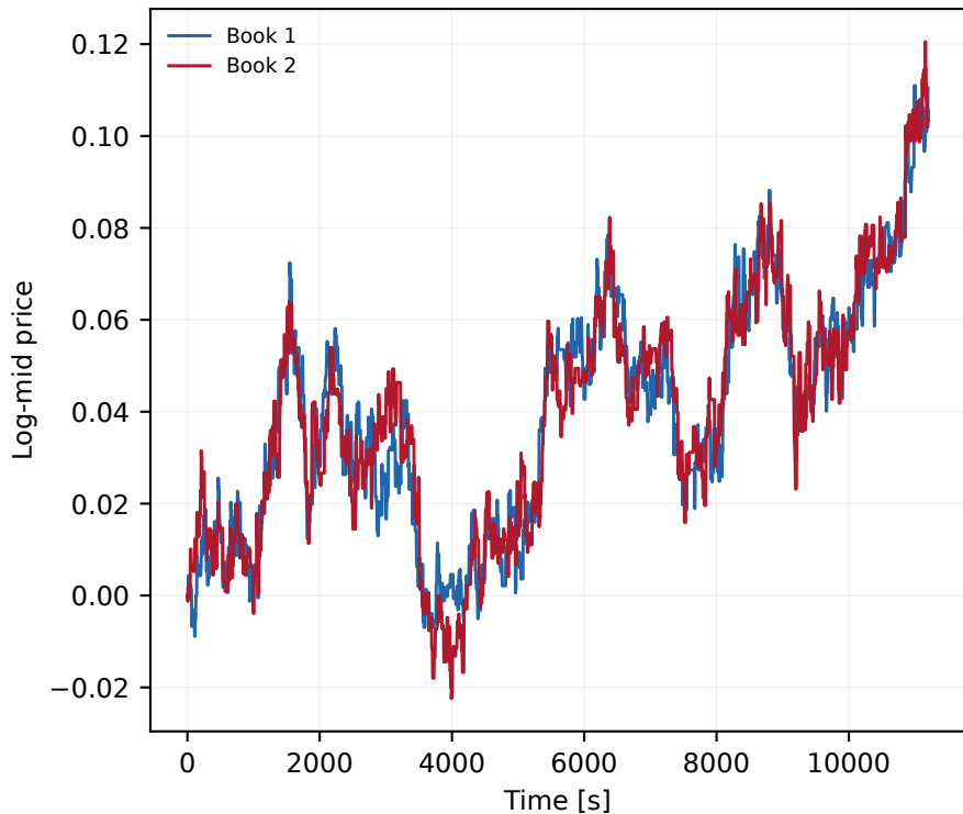
(d) Poisson: price path
