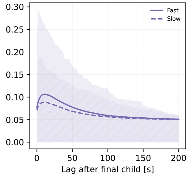
Mittag-Leffler
