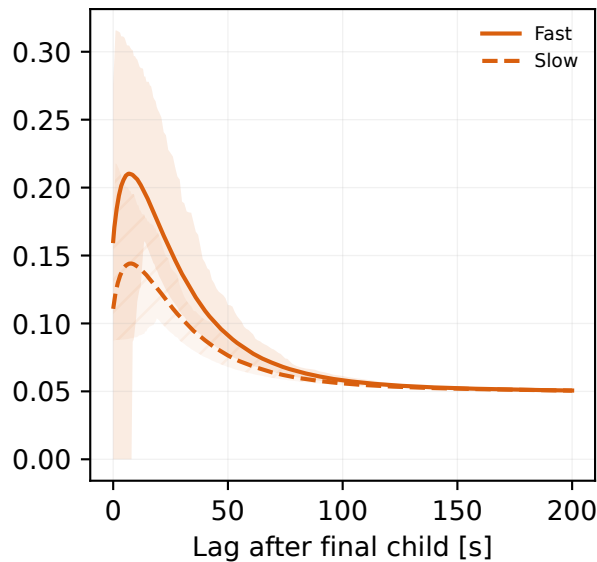
Poisson
