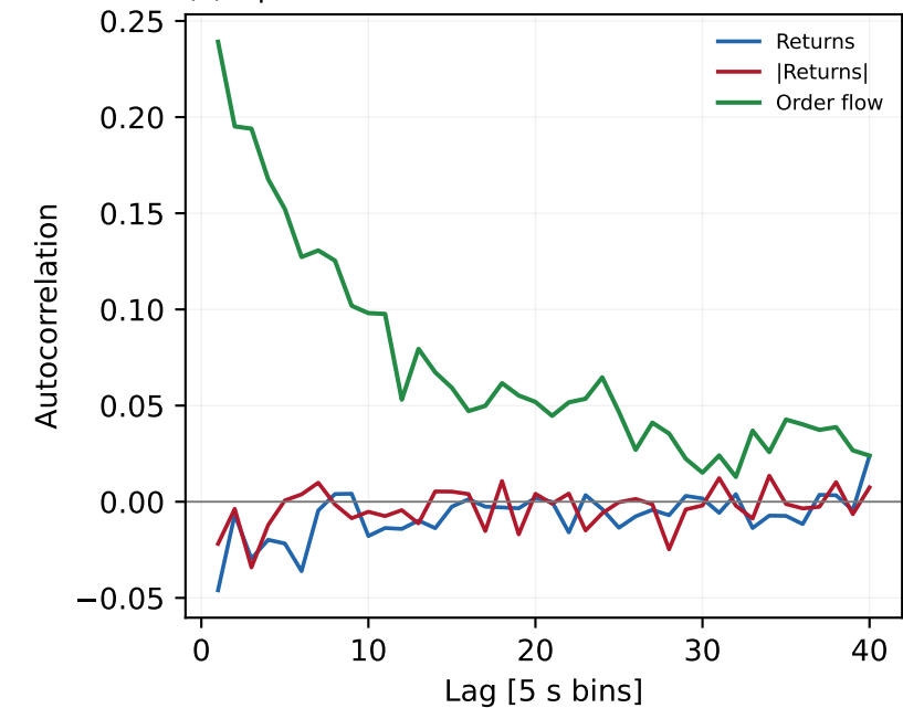
(f) Poisson: acf
