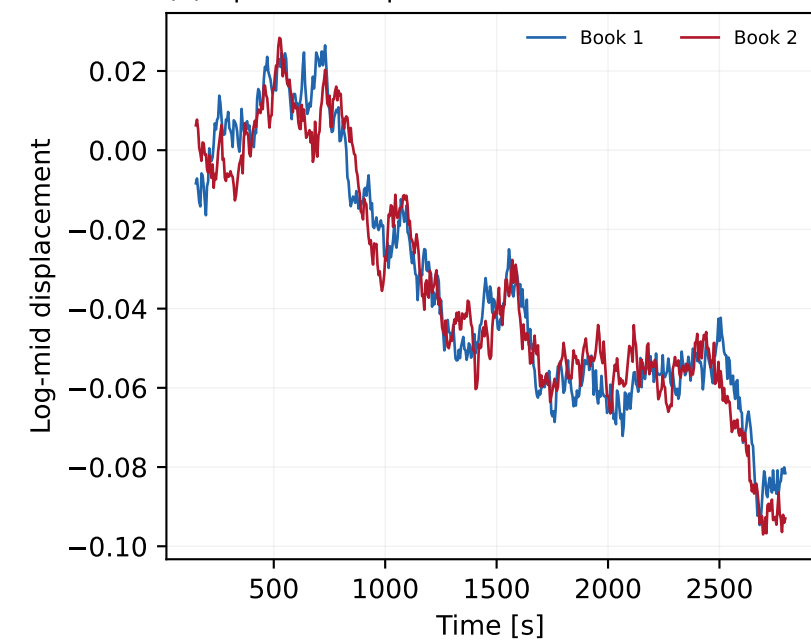
(d) Poisson: price returns
