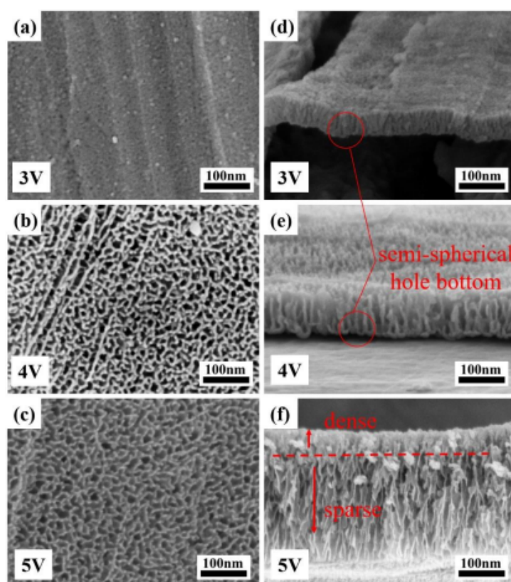
图 2.1 阳极氧化锡在 0.25M NaOH 中，在 3V（a，d），4V（b，e）和 5V（c，f）下阳极氧化 10min 后的 SEM 图像，俯视图（a-c）和横断面图（d-f）
