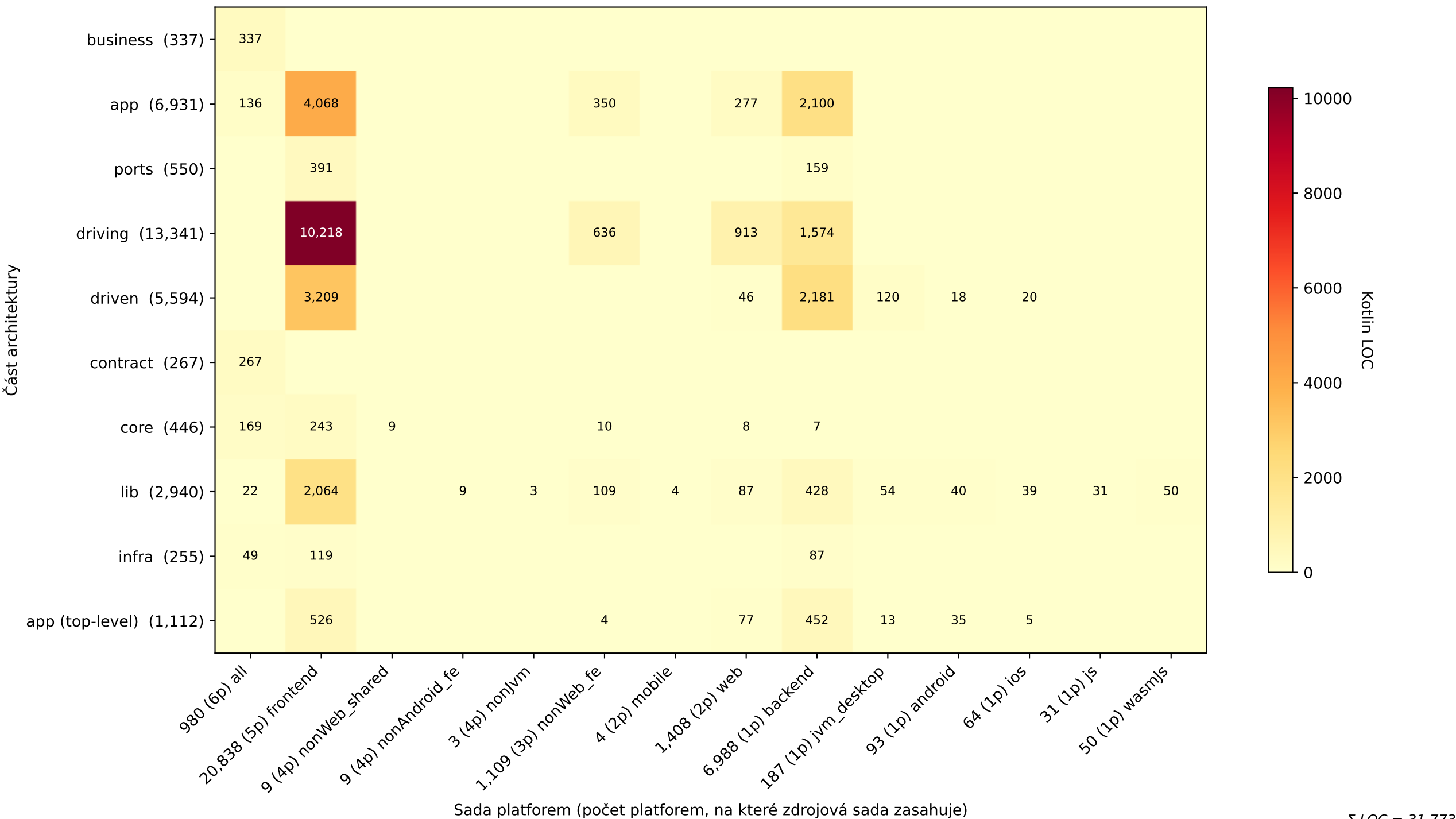
Rozdělení kódu dle zdrojových sad a částí architektury
