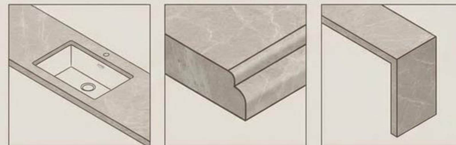
ВЫРЕЗ ПОД МОЙКУ
