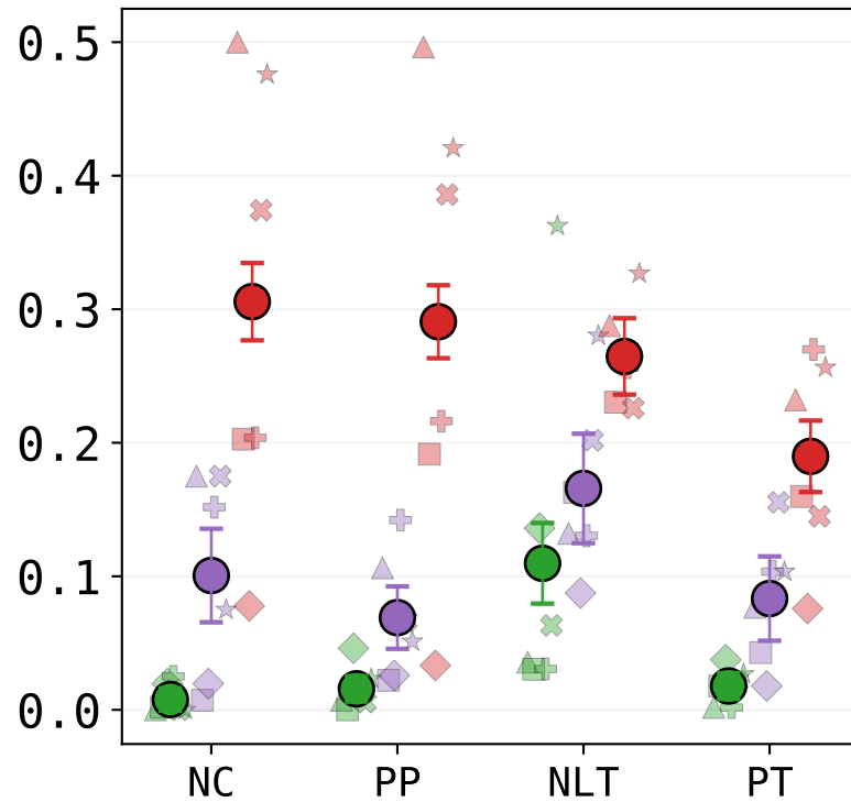
Gini
