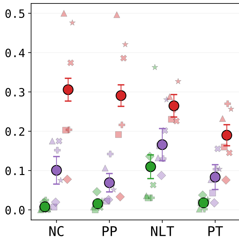
Gini
