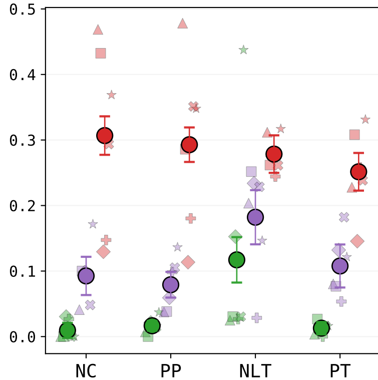
Gini
