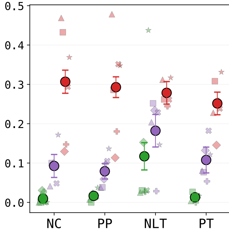
Gini
