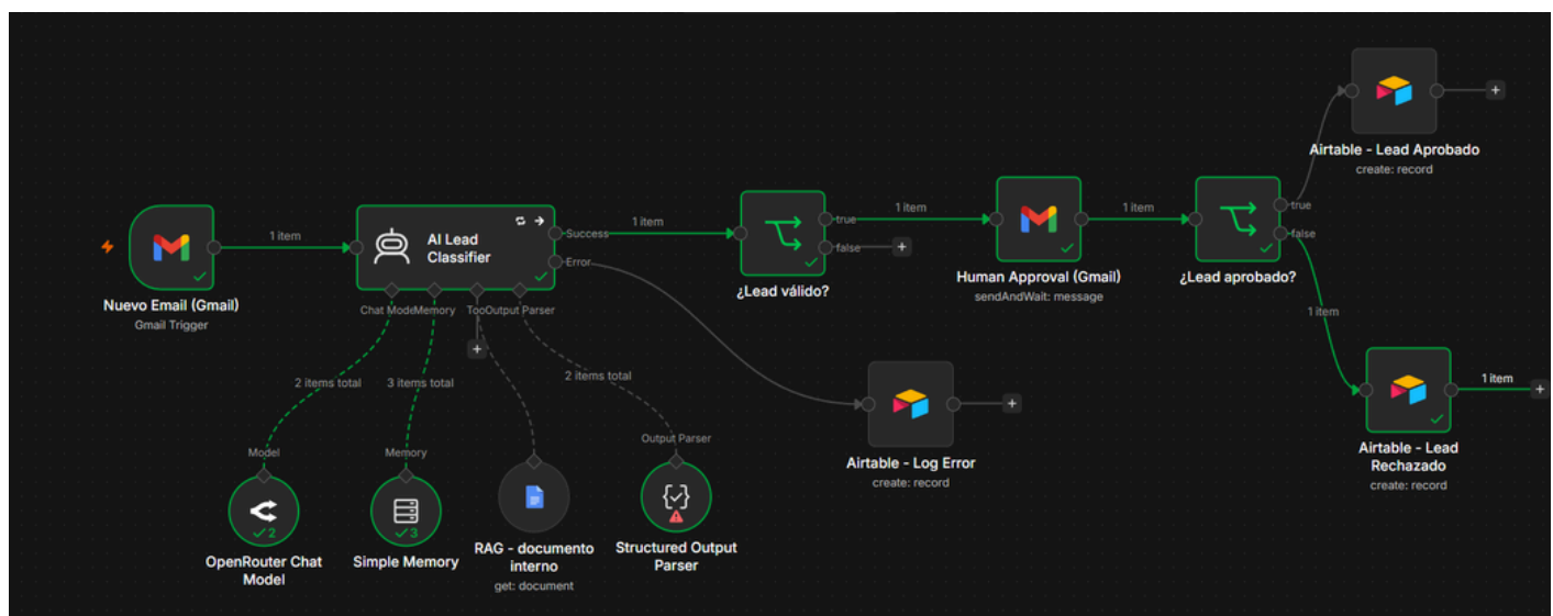
Figura 5. Ejecución del flujo mostrando el recorrido completo de los nodos y la correcta comunicación entre Gmail, el Agente de IA y Airtable.
