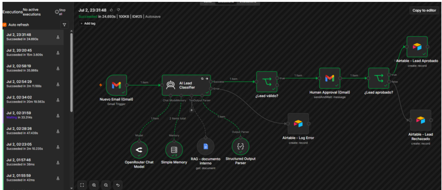
Figura 4. Ejecución exitosa del flujo principal en n8n. Se observa el procesamiento automático del correo electrónico, la clasificación mediante IA, la validación humana y el registro del resultado.
