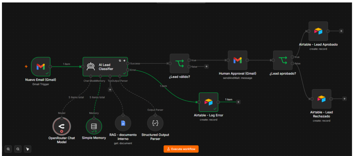
Figura 8. Ejecución del flujo utilizando la ruta de error, registrando automáticamente la incidencia en Airtable.
