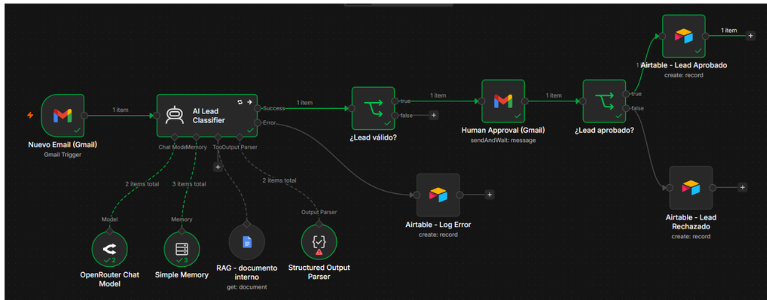
Figura 2. Flujo principal implementado en n8n.
