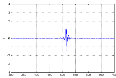
Рисунок 3: Экспериментально полученная интерферограмма для стекла
