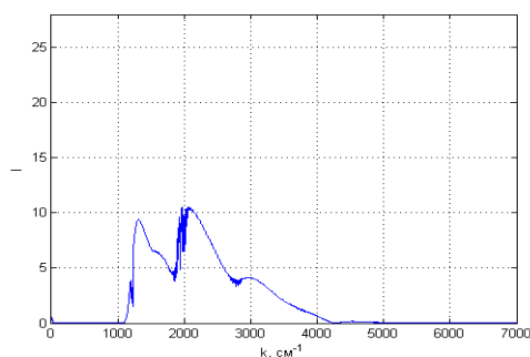
Рисунок 6: ПФ интерферограммы для стекла
