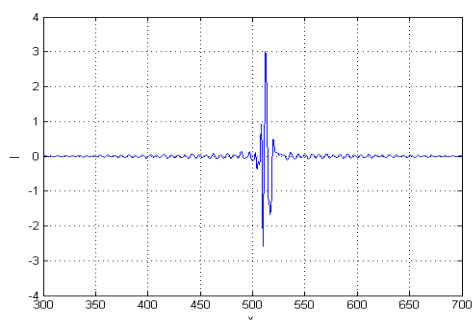
Рисунок 2: Экспериментально полученная интерферограмма для пустого канала
