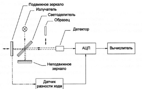
Рисунок 1: Схема устройства Фурье-интерферометра
