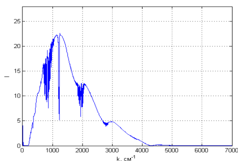
Рисунок 5: ПФ интерферограммы для пустого канала
