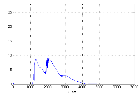
Рисунок 7: ПФ интерферограммы для стекла с напылением CuO
