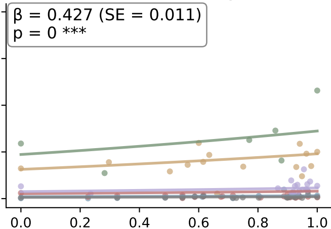
CanaryV2
