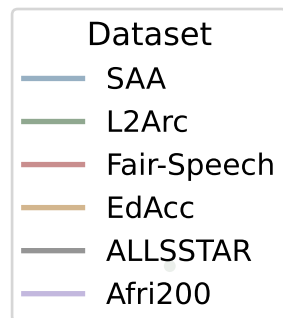
CanaryV2
