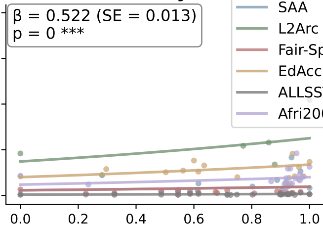
CanaryV2
