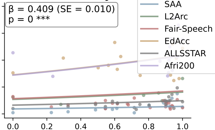
CanaryV2
