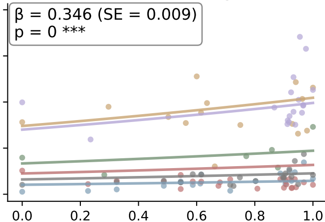
CanaryV2
